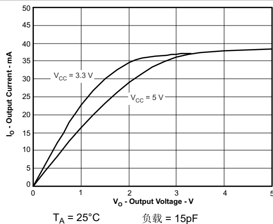
图 5-10. 低电平输出电流与低电平输出电压间的关系
