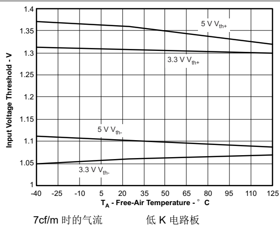
图 5-7. 输入电压阈值与自然通风条件下的温度间的关系
