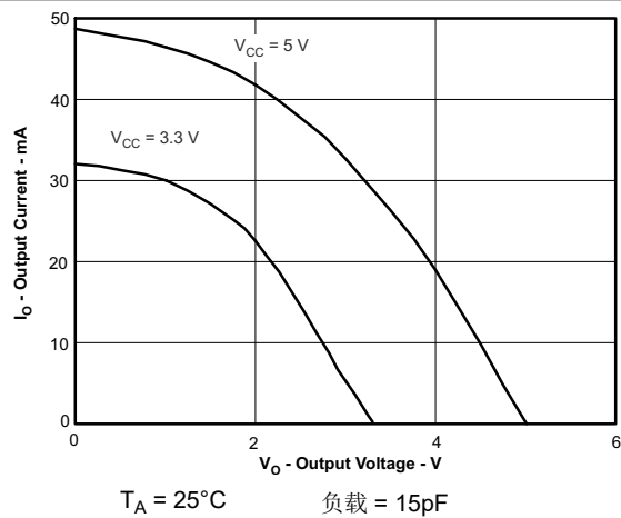
图 5-9. 高电平输出电流与高电平输出电压间的关系
