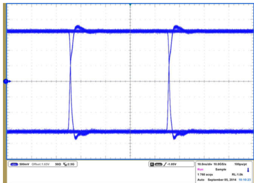
图 8-6. 25Mbps、3.3V 和 25°C 下的 ISO7242M 眼图
