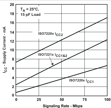
图 5-2. 3.3V RMS 电源电流与信号传输速率 (Mbps) 间的关系
