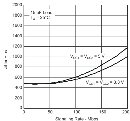
图 5-13. ISO722xM 抖动与信令速率间的关系
