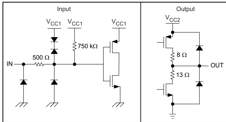
图 7-1. 器件 I/O 原理图
