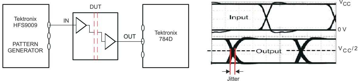
图 6-4. 峰值间眼图抖动测试电路和电压波形
