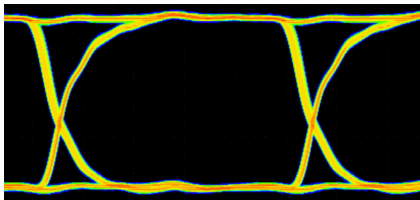
图 9-4. 100Mbps PRBS 2^{16} - 1、3.3V 和 25°C 下的 ISO643x-Q1 眼图
