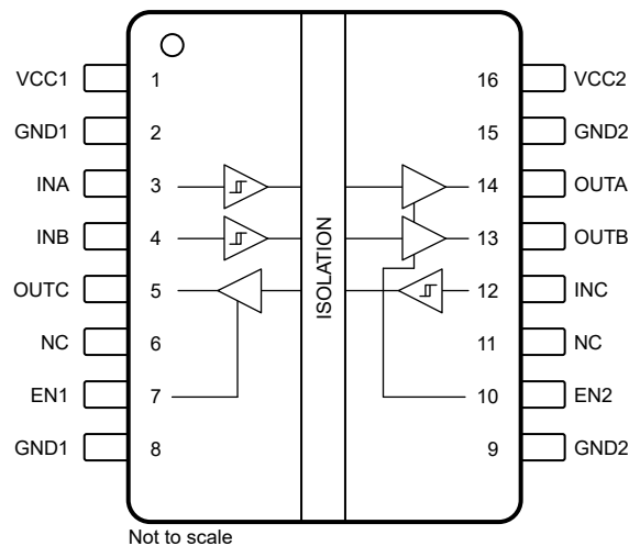
图 5-1. ISO6431-Q1 和 ISO6431F-Q1 顶视图
