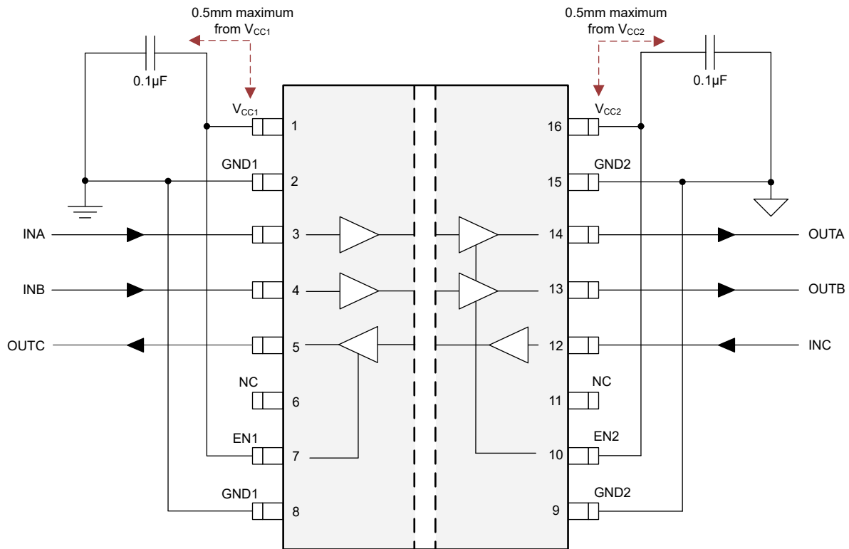
图 9-2. 典型 ISO643x-Q1 电路
