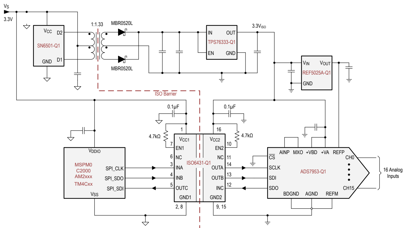
图 9-1. 3 通道典型应用
