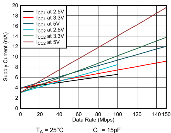
图 6-7. ISO6431-Q1 或 ISO6431F-Q1 电源电流与数据速率间的关系 (15pF 负载)
