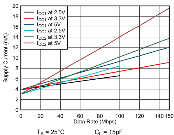
图 6-7. ISO6431 或 ISO6431F 电源电流与数据速率间的关系 (15pF 负载)
