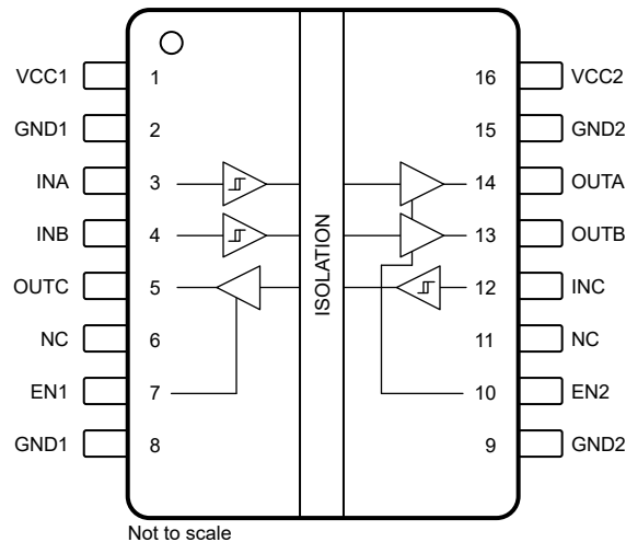
图 5-1. ISO6431 和 ISO6431F 顶视图
