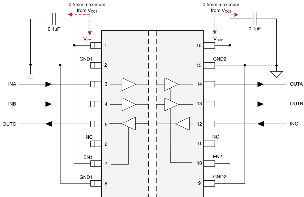
图 9-2. 典型 ISO643x 电路
