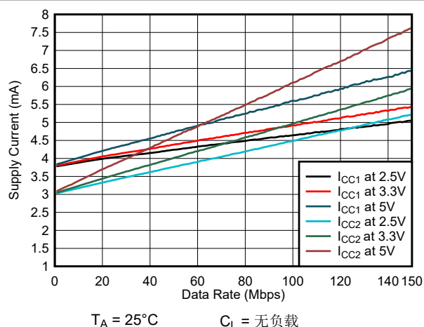
图 6-8. ISO6431 或 ISO6431F 电源电流与数据速率间的关系 (无负载)
