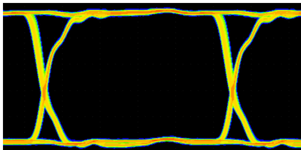
图 9-3. 100Mbps PRBS 2^{16} - 1、5V 和 25°C 下的 ISO643x 眼图
