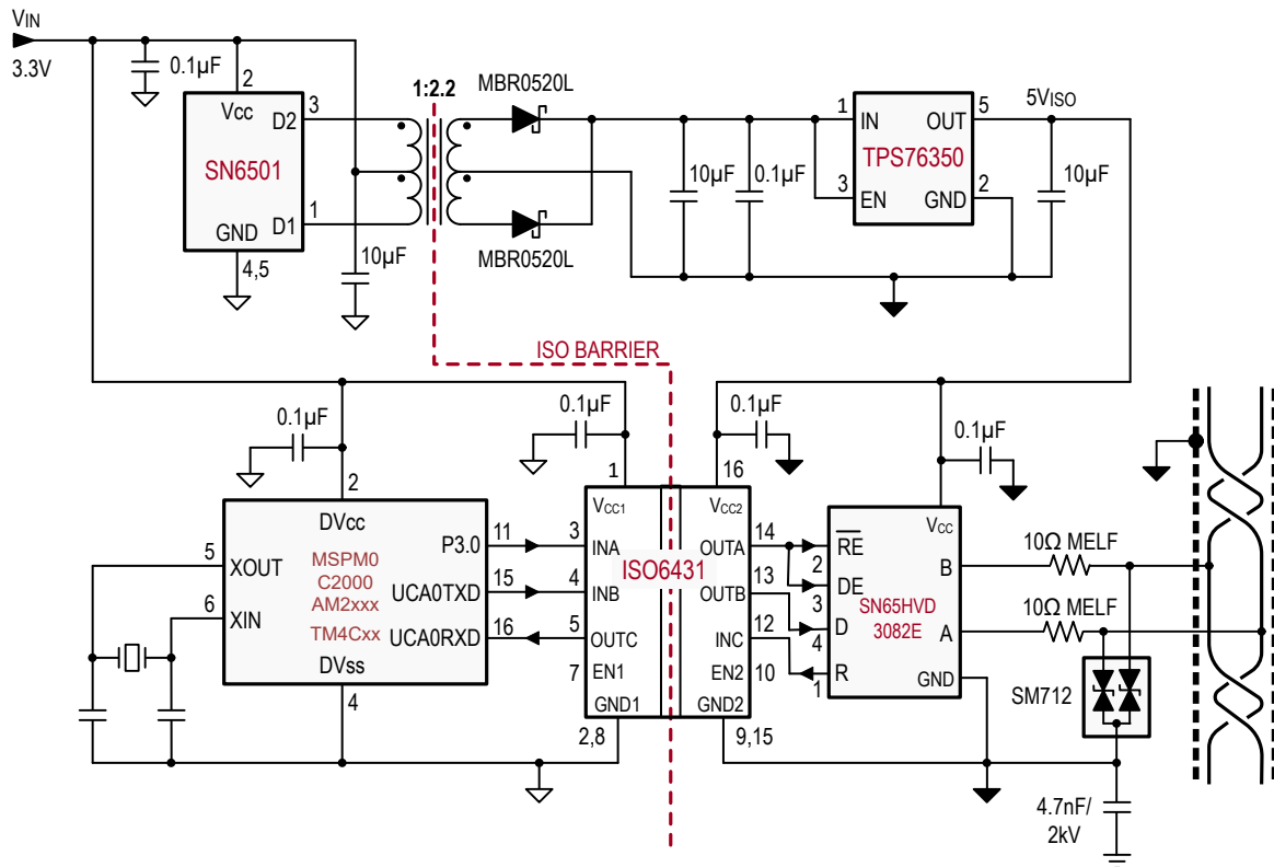
图 9-1. 3 通道典型应用
