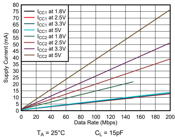
图 6-7. ISO6040H 或 ISO6040L 电源电流与数据速率间的关系 (15pF 负载)
