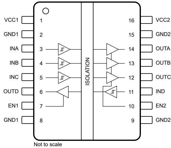
图 5-2. ISO6041H 和 ISO6041L 顶视图
