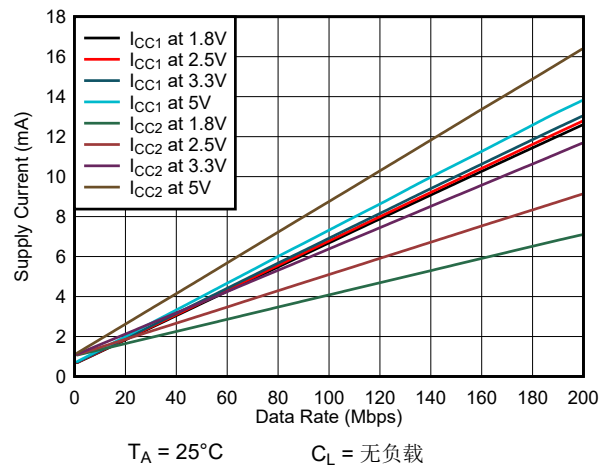
图 6-8. ISO6040H 或 ISO6040L 电源电流与数据速率间的关系 (无负载)
