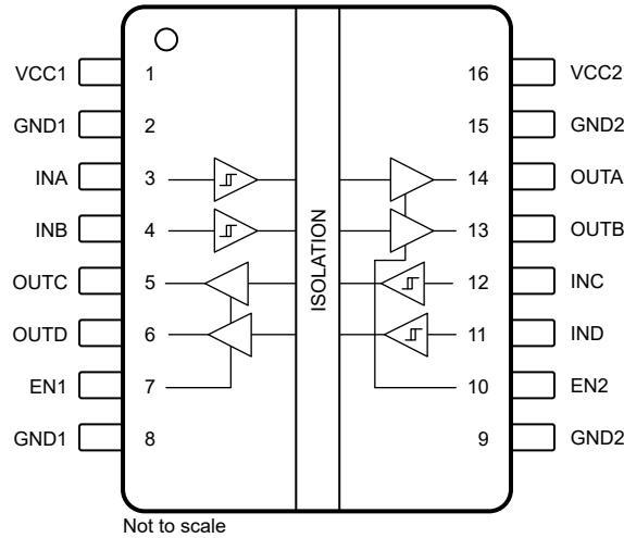
图 5-3. ISO6042H 和 ISO6042L 顶视图
