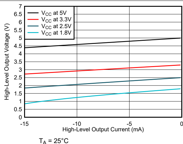
图 6-13. 高电平输出电压与高电平输出电流间的关系
