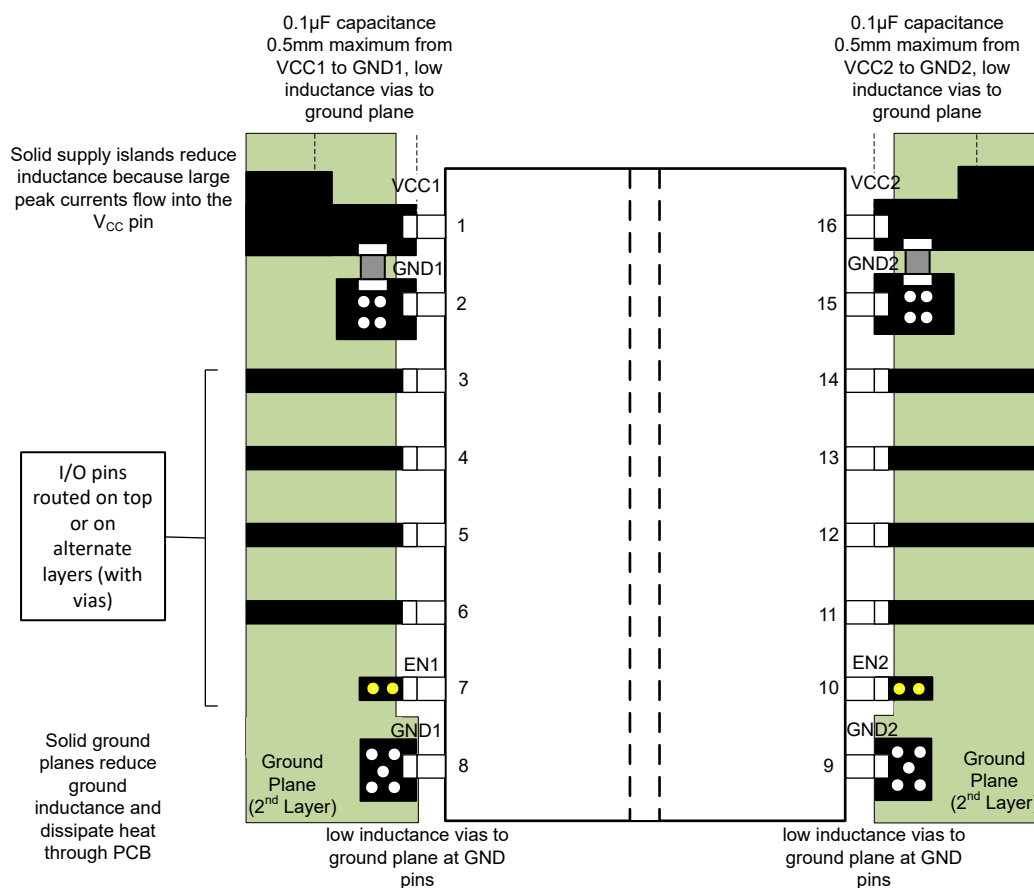
图 9-8. 布局示例
