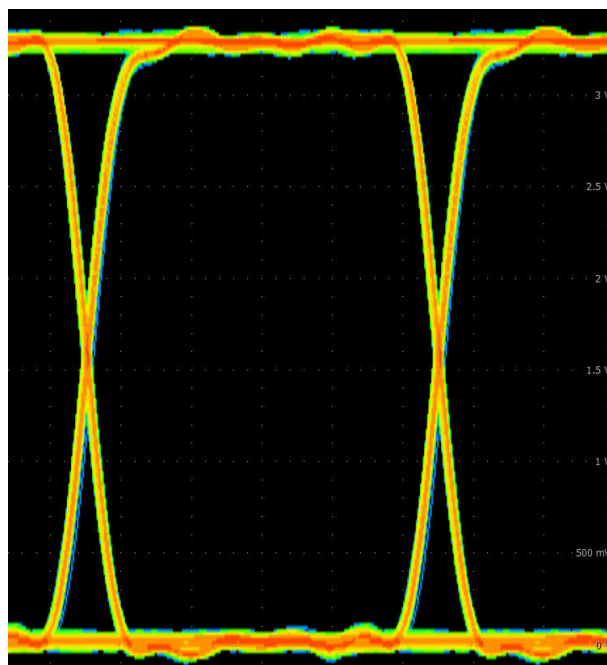
图 9-5. 200Mbps PRBS 2 16 - 1、3.3V 和 25°C 下的 ISO604x 眼图
