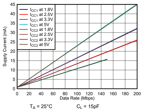
图 6-11. ISO6042H 或 ISO6042L 电源电流与数据速率间的关系 (15pF 负载)
