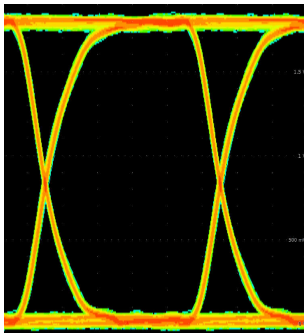
图 9-7. 200Mbps PRBS 2^{16} - 1、1.8V 和 25°C 下的 ISO604x 眼图
