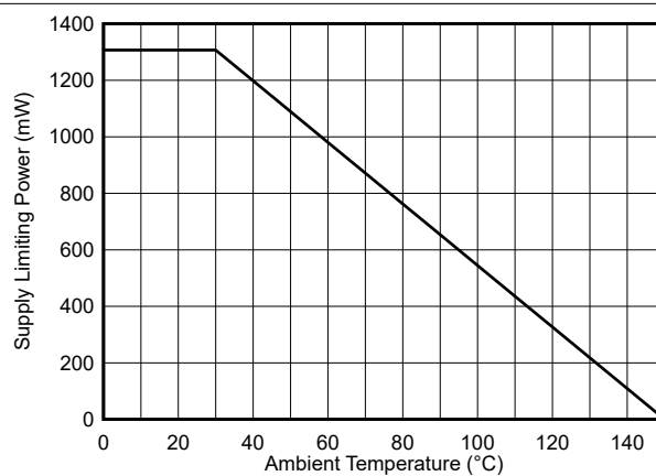
图 6-6. SSOP (DBQ-16) 封装安全限制功率的热降额曲线
