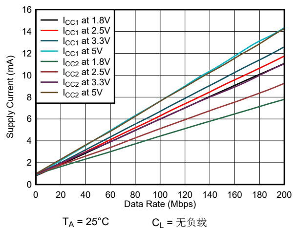
图 6-10. ISO6041H 或 ISO6041L 电源电流与数据速率间的关系 (无负载)
