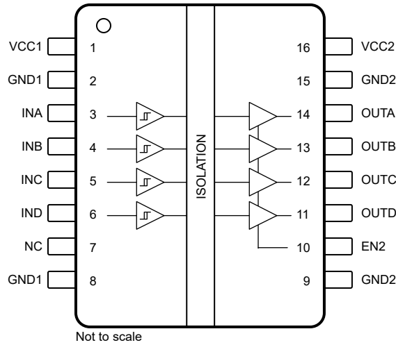
图 5-1. ISO6040H 和 ISO6040L 顶视图
