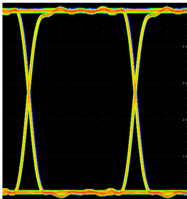
图 9-4. 200Mbps PRBS 2 16 - 1、5V 和 25°C 下的 ISO604x 眼图
