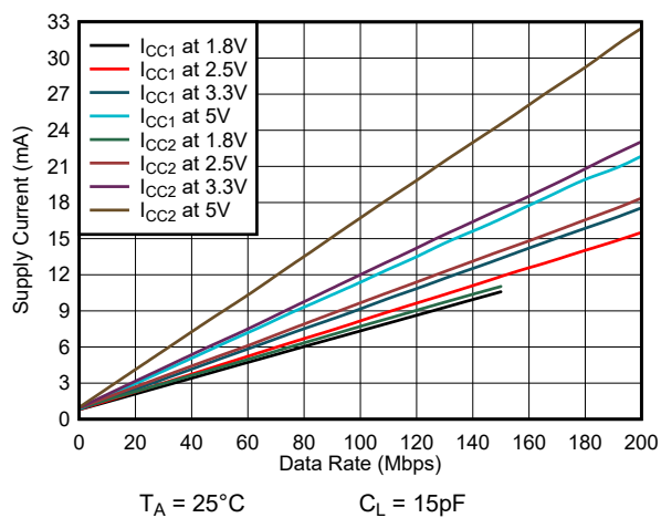
图 6-9. ISO6041H 或 ISO6041L 电源电流与数据速率间的关系 (15pF 负载)
