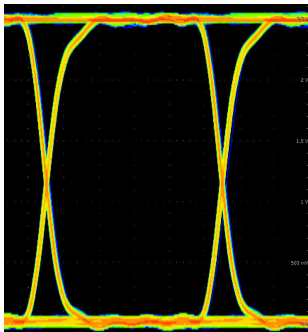
图 9-6. 200Mbps PRBS 2^{16} - 1、2.5V 和 25°C 下的 ISO604x 眼图
