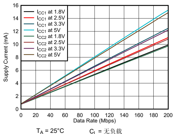
图 6-12. ISO6042H 或 ISO6042L 电源电流与数据速率间的关系 (无负载)
