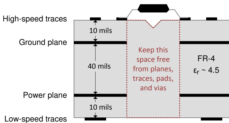
图 9-9. 布局示例 PCB 横截面
