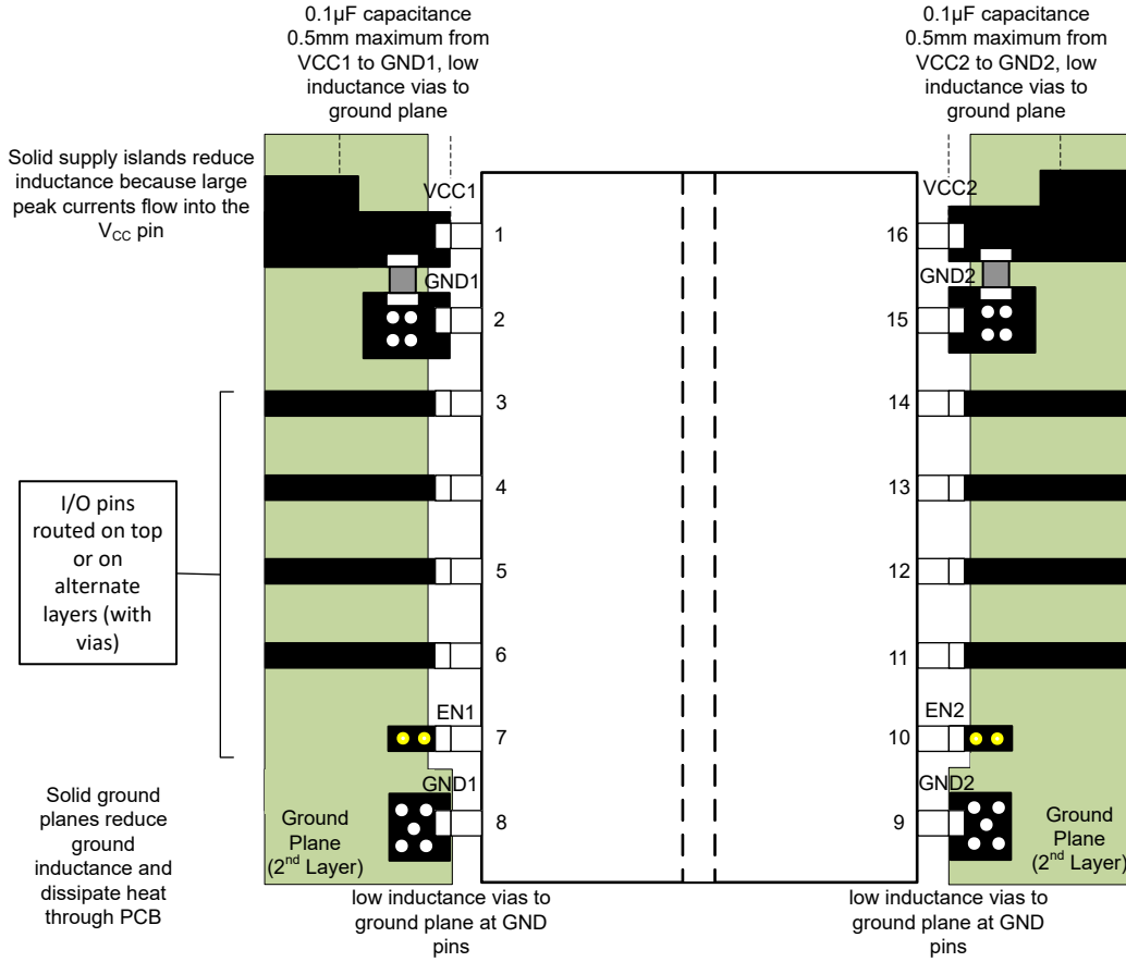
图 9-4. 布局示例
