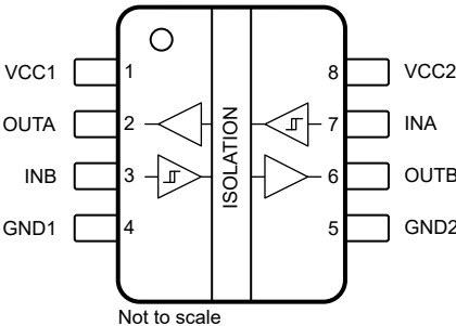
图 5-2. ISO6021H 和 ISO6021L 顶视图
