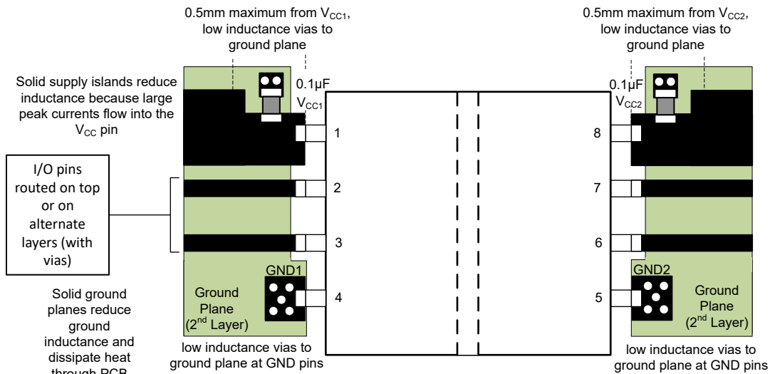
图 9-3. 布局示例
