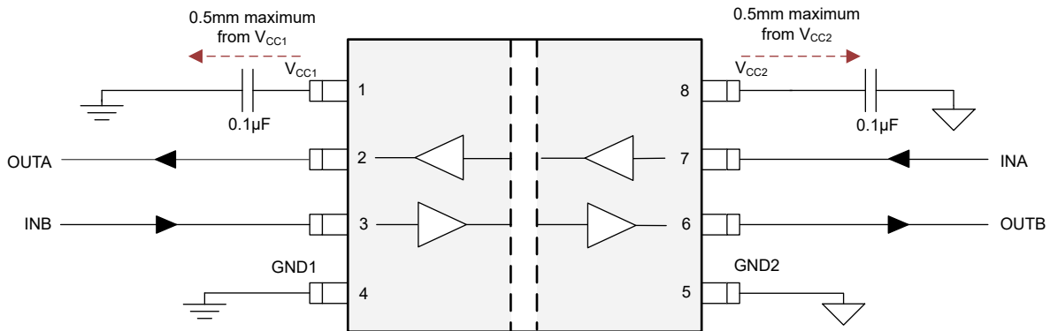
图 9-2. 典型 ISO602x 电路
