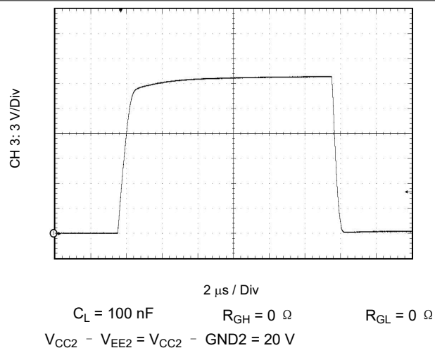
图 7-11. Output Transient Waveform
