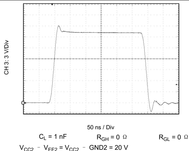
图 7-9. Output Transient Waveform
