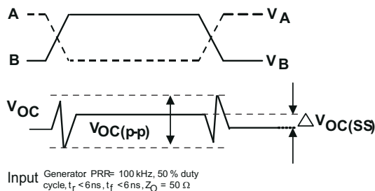
图 7-3. 驱动器共模输出电压的测试电路和波形定义
