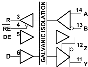
图 8-1. ISO3080、IOS3086 功能图
