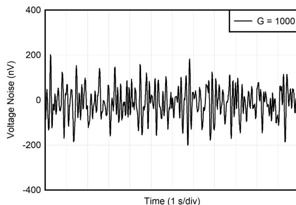
图 7-28. 0.1-Hz to 10-Hz RTI Voltage Noise
