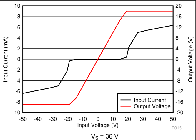
图 7-16. Input Current vs Input Overvoltage
