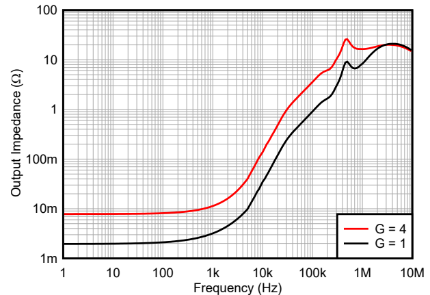
图 5-30. 输出阻抗与频率间的关系
