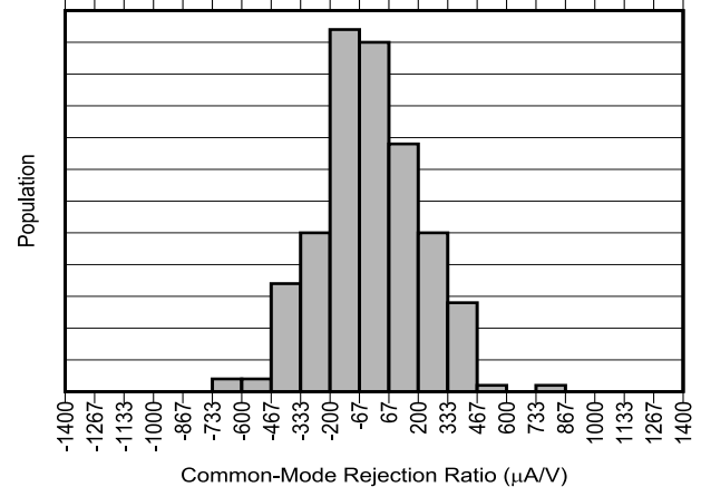
图 5-6. INA790B 共模抑制产生分布图
