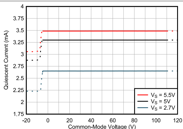
图 5-24. 静态电流与共模电压间的关系
