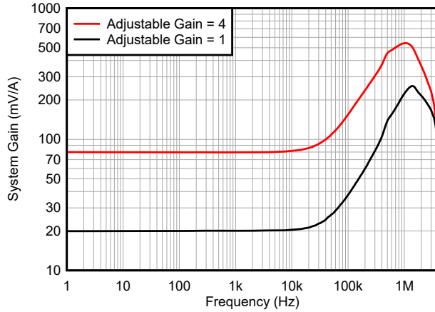
图 5-27. 系统增益与频率间的关系
