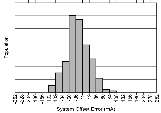
图 5-2. INA790B 输入失调电流产生分布图
