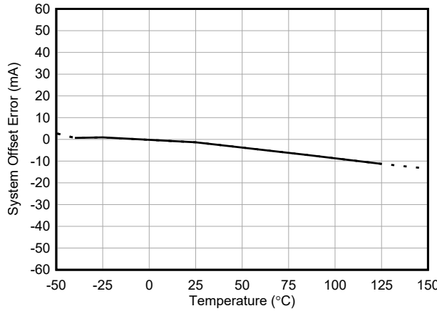
图 5-3. INA790A 输入失调电流与温度间的关系
