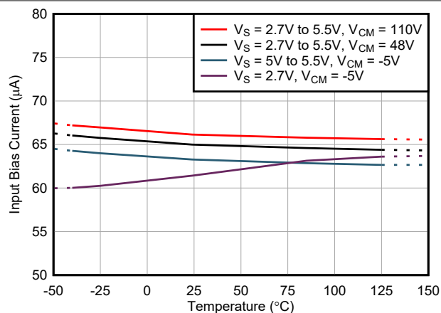
图 5-21. 总输入偏置电流与温度间的关系
