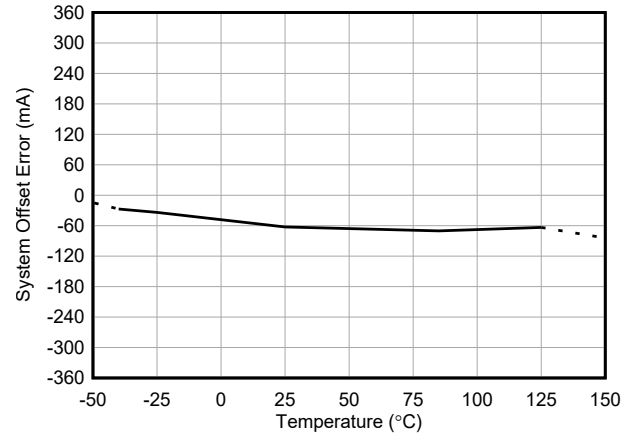
图 5-4. INA790B 输入失调电流与温度间的关系
