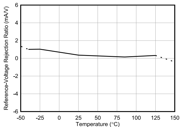
图 5-9. 基准电压抑制比与温度间的关系
