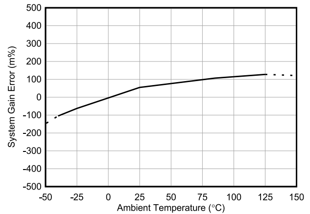
图 5-14. INA790B 增益误差与温度间的关系
