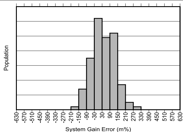
图 5-12. INA790B 增益误差产生分布图
