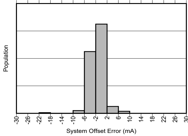
图 5-1. INA790A 输入失调电流产生分布图
