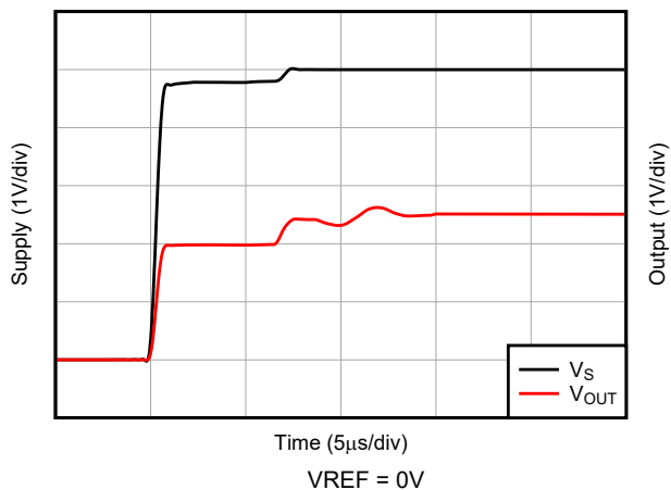
图 5-35. 启动响应
