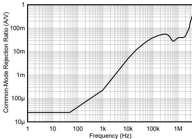
图 5-29. 共模抑制比与频率间的关系
