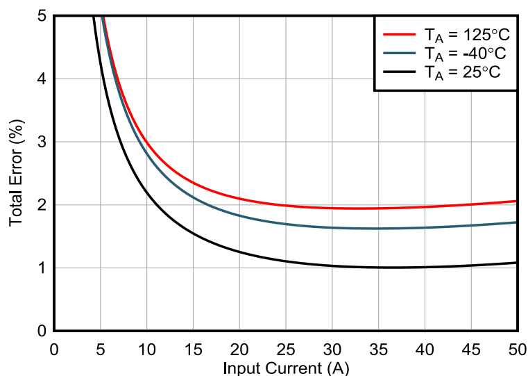
图 7-1. INA790A 总误差与输入电流间的关系
