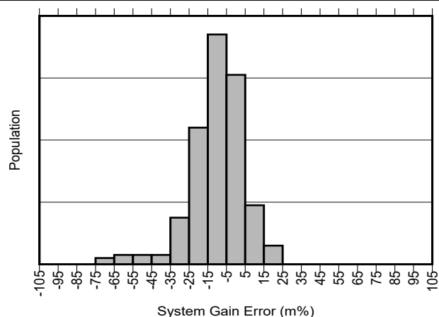
图 5-11. INA790A 增益误差产生分布图
