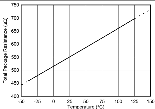
图 5-19. 封装电阻与温度间的关系
