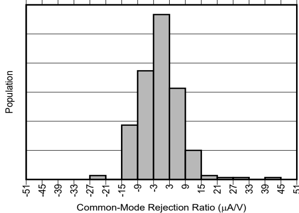
图 5-5. INA790A 共模抑制产生分布图
