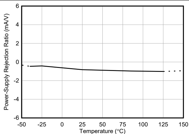
图 5-8. 电源抑制比与温度间的关系
