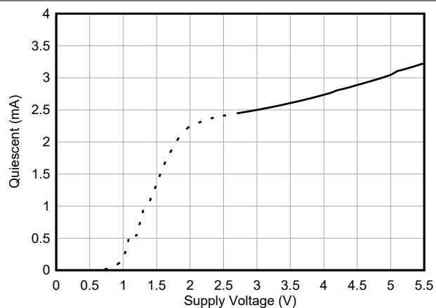
图 5-22. 静态电流与电源电压间的关系
