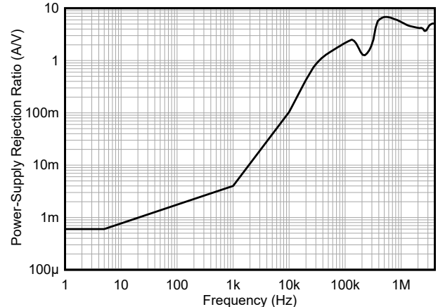
图 5-28. 电源抑制比与频率间的关系
