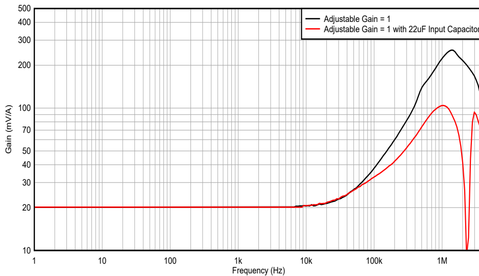
图 7-4. 添加 22μF 输入电容器之前和之后 INA790x 增益与频率间的关系
