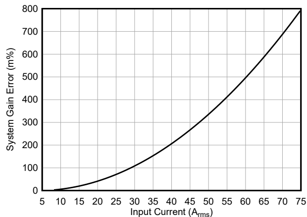
图 5-10. 系统增益误差与输入电流间的关系
