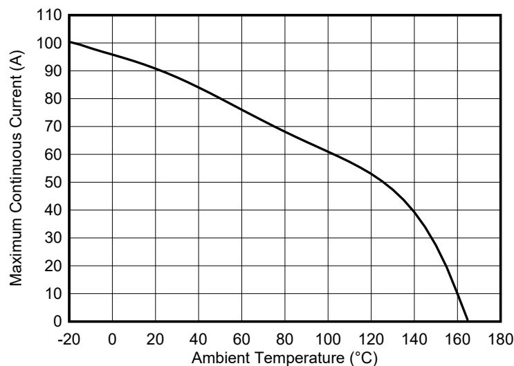
图 6-2. 最大连续电流与环境温度间的关系
