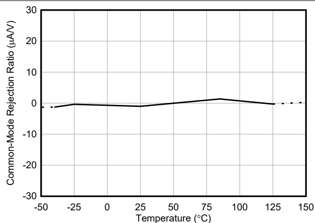
图 5-7. 共模抑制比与温度间的关系
