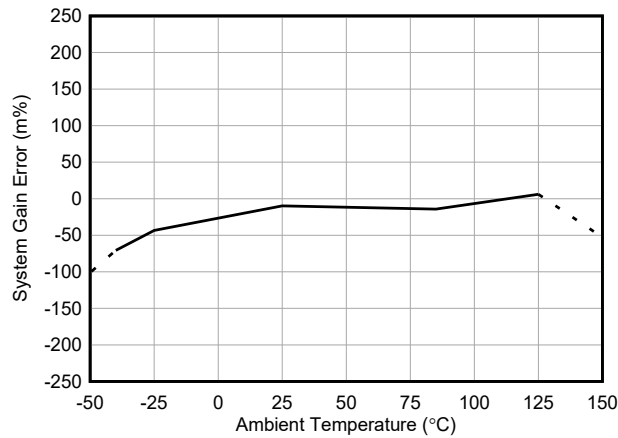
图 5-13. INA790A 增益误差与温度间的关系
