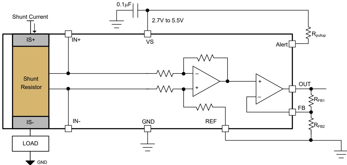
图 6-5. 以接地为基准的输出
