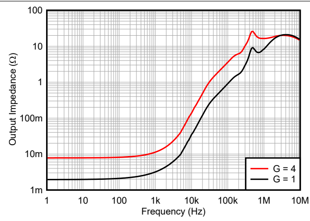
图 5-30. 输出阻抗与频率间的关系
