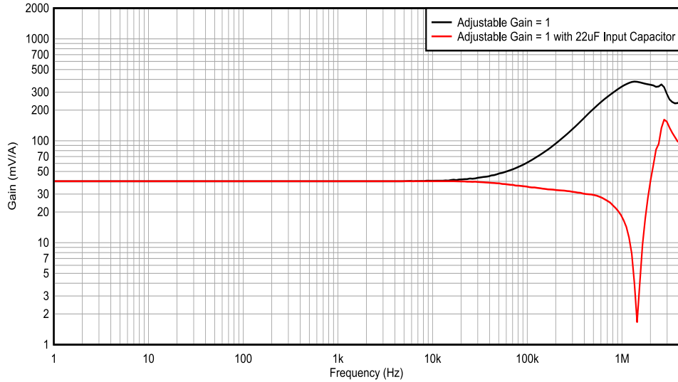
图 7-4. 添加 22 \mu F 输入电容器之前和之后 INA750x-Q1 增益与频率间的关系
