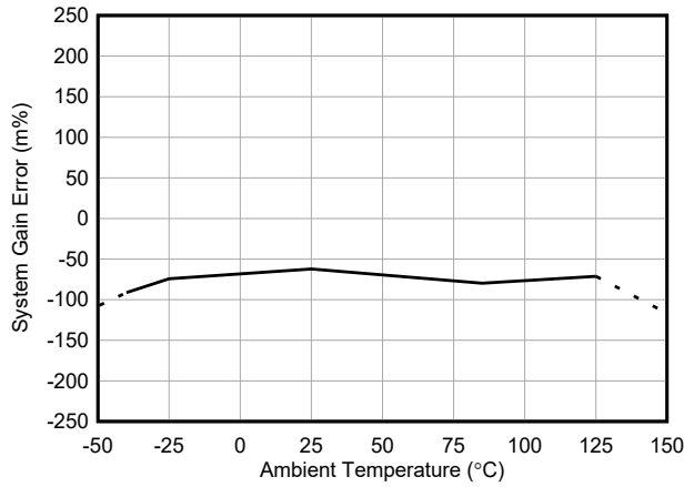
图 5-13. INA750A-Q1 增益误差与温度间的关系
