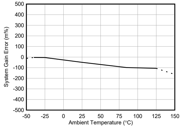
图 5-14. INA750B-Q1 增益误差与温度间的关系
