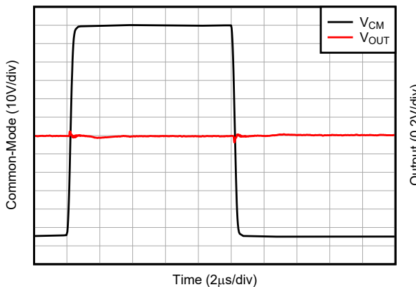
图 5-34. 共模瞬态响应
