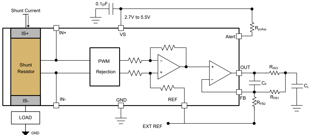
图 7-5. 具有 RISO 双反馈的 INA750x-Q1
