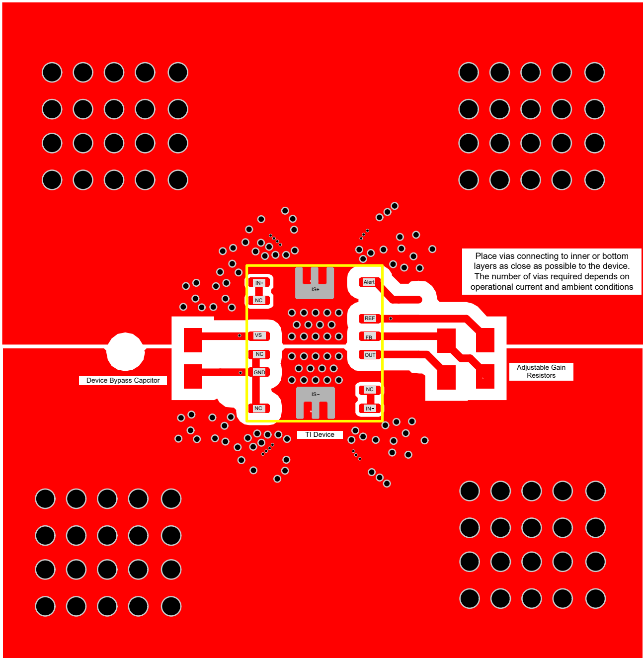
图 7-12. INA750x-Q1 布局示例
