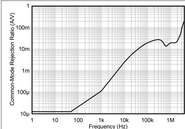
图 5-29. 共模抑制比与频率间的关系
