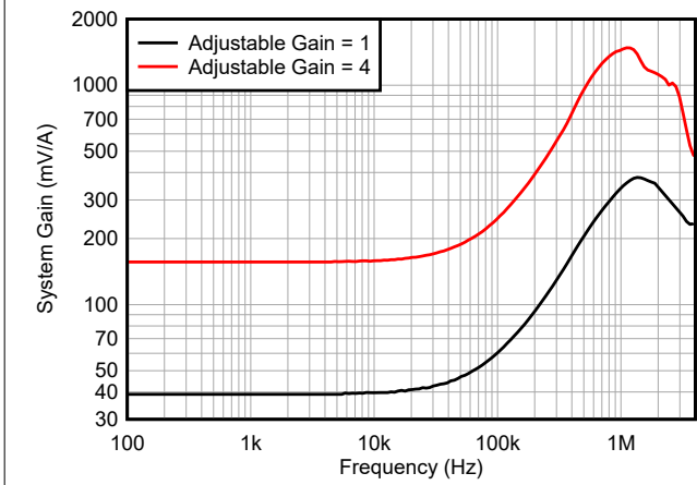
图 5-27. 系统增益与频率间的关系
