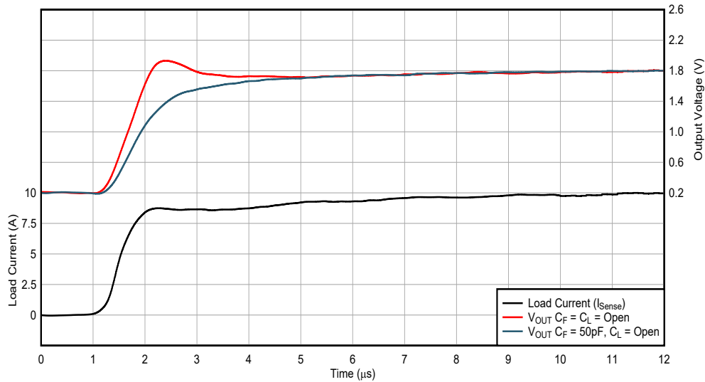
图 7-6. 可调增益为 1 时 RISO 双反馈前后的 INA750x-Q1 负载阶跃响应
