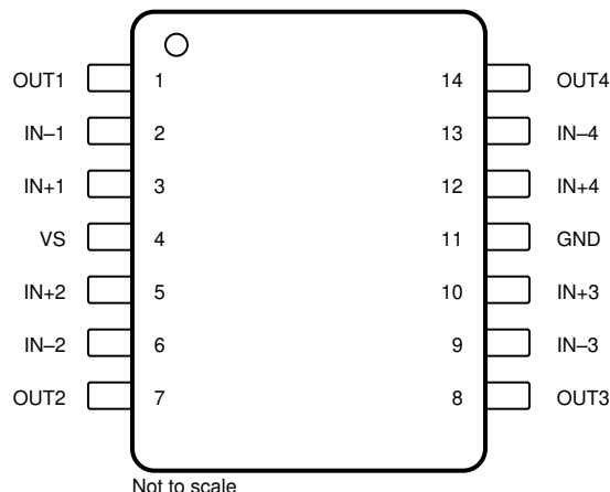
图 6-4. INA4180-Q1 : PW 封装 14 引脚 TSSOP 顶视图
