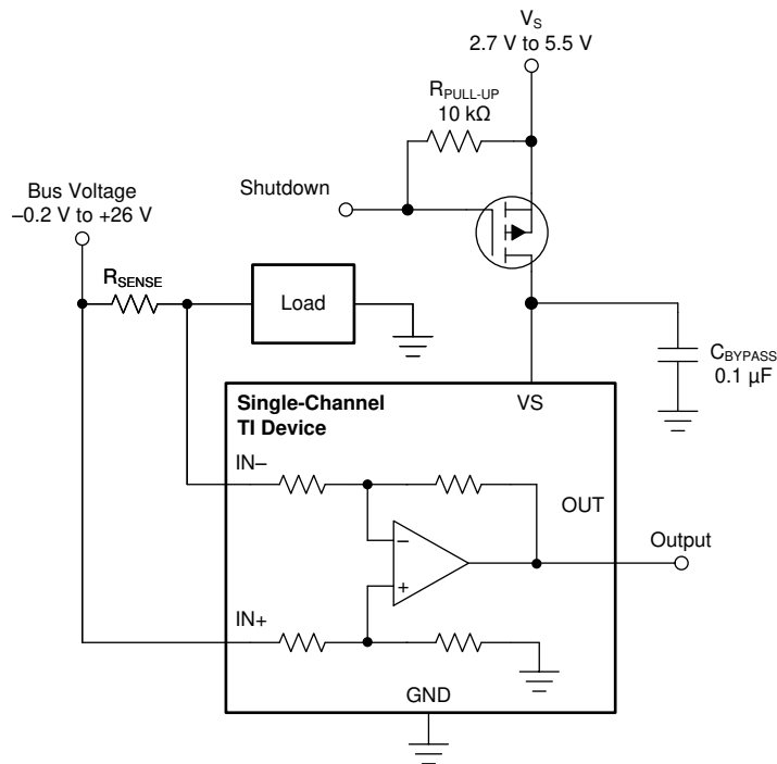
图 8-6. 关断 INxA180-Q1 的基本电路
