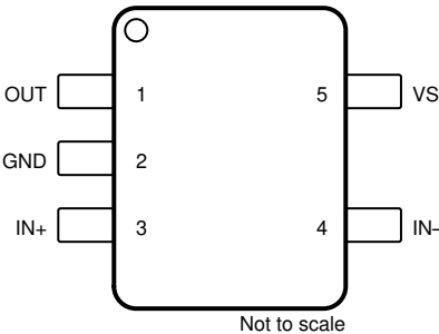
图 6-1. INA180 : DBV 封装 5 引脚 SOT-23 ( 引脚排列 A ) 顶视图
