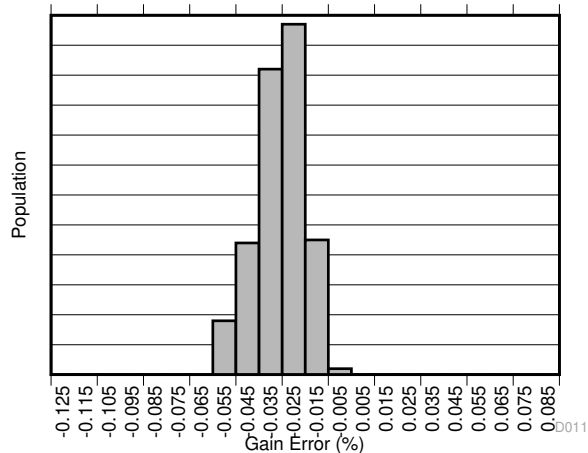
图 6-11. 增益误差产生分布图 (INA381A1-Q1)
