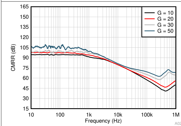
图 7-29. CMRR (以输入为参考) 与频率间的关系
