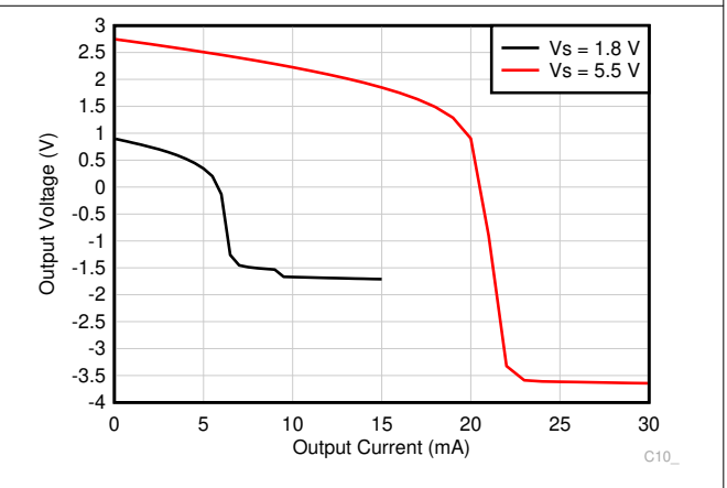
图 7-26. 输出电压与输出电流 (拉电流) 间的关系
