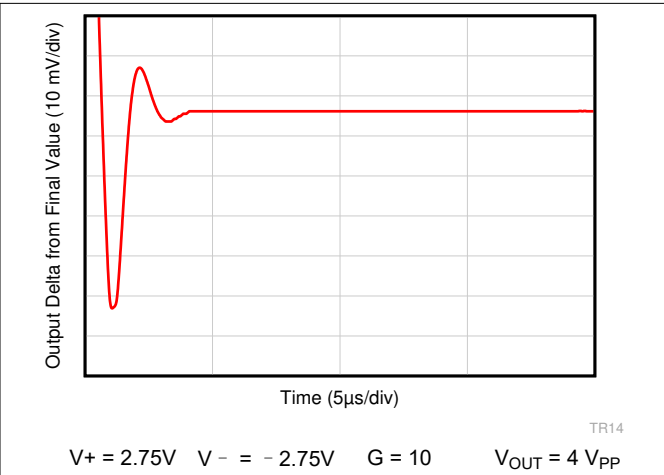
图 7-42. 大信号稳定时间 (下降沿)
