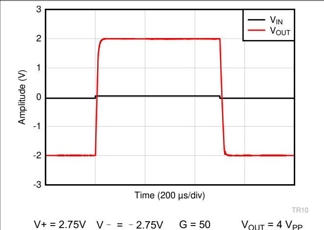
图 7-44. 大信号阶跃响应
