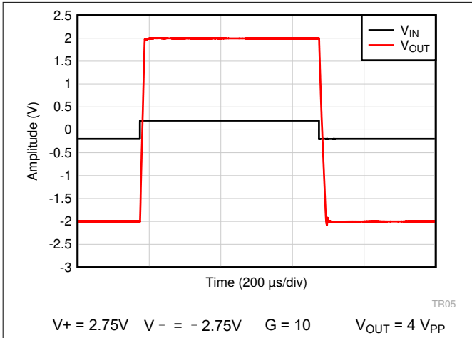
图 7-41. 大信号阶跃响应
