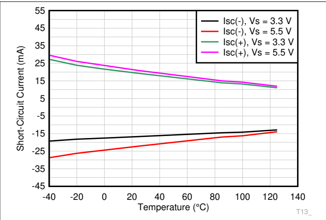
图 7-16. 短路电流与温度间的关系
