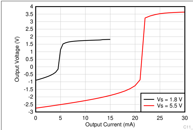
图 7-27. 输出电压与输出电流 (灌电流) 间的关系
