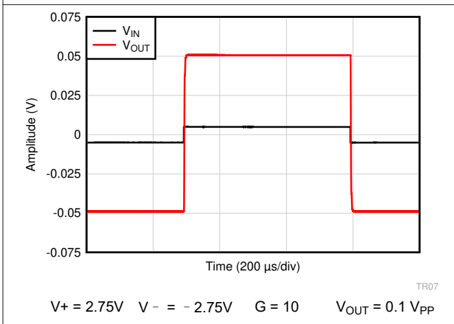
图 7-45. 小信号阶跃响应
