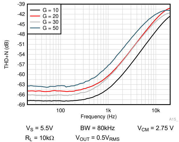
图 7-36. THD + N 与频率间的关系
