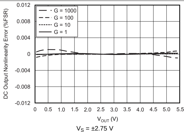
图 9. Nonlinearity Error
