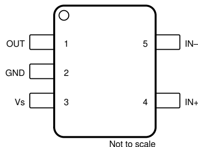
图 5-2. INA281B-Q1 : DBV 封装 5 引脚 SOT-23 顶视图
