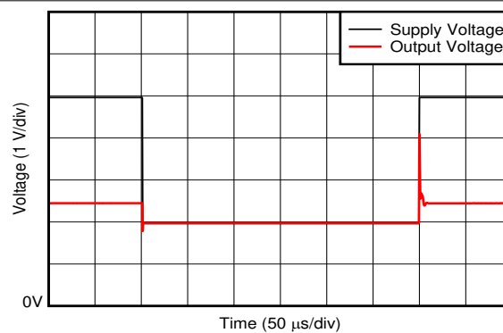
图 7-26. 电源瞬态响应
