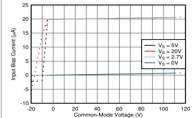
图 5-5. 输入偏置电流与共模电压间的关系 V_{\text{SENSE}} = 0\text{V}
