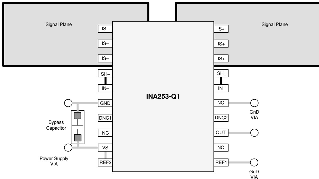
图 10-1. INA253-Q1 Layout Example
