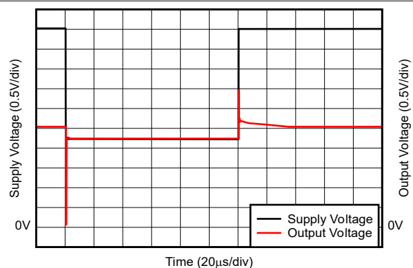
图 6-37. 欠压恢复
