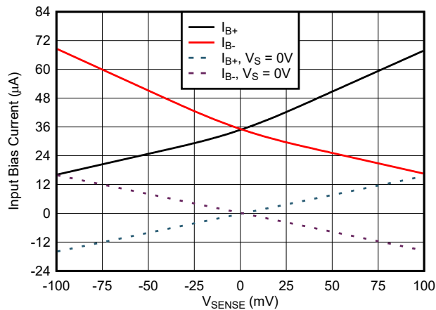
图 6-19. INA241x2 输入偏置电流与 V_{\text{SENSE}} 间的关系
