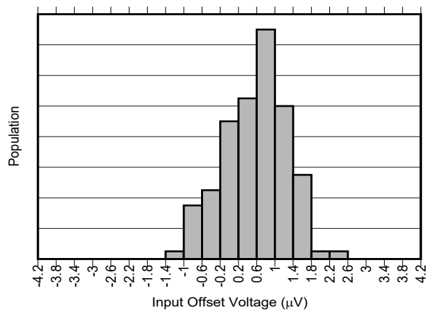
图 6-4. INA241A5 输入失调电压产生分布图
