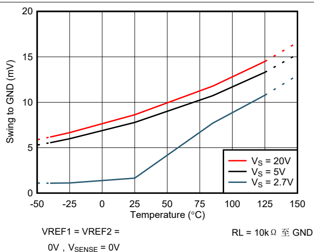
图 6-26. 相对于 GND 的摆幅与温度间的关系
