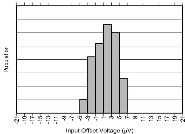
图 6-1. INA241A1 输入失调电压产生分布图
