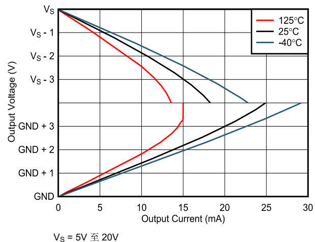
图 6-23. 输出电压与输出电流间的关系
