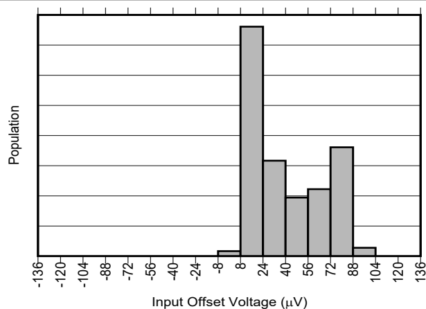
图 6-3. INA241A3 和 INA241A4 输入失调电压产生分布图
