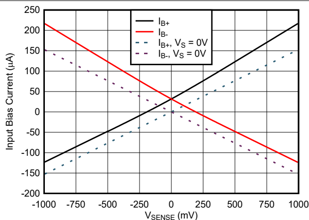
图 6-19. INA241x2 输入偏置电流与 V_{\text{SENSE}} 间的关系
