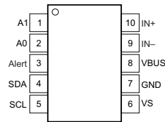
图 5-2. DGS Package 10-Pin VSSOP (Top View)
