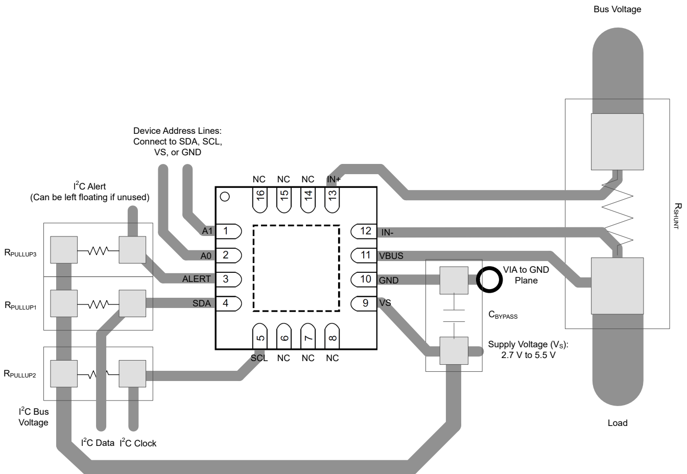
图 8-4. Layout Example (RGT Package)
