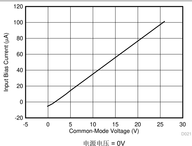
图 6-21. 输入偏置电流与共模电压间的关系 (两种输入, 关断)
