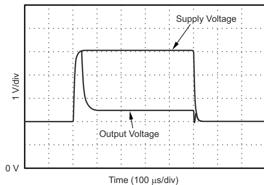
图 7-19. 欠压恢复
