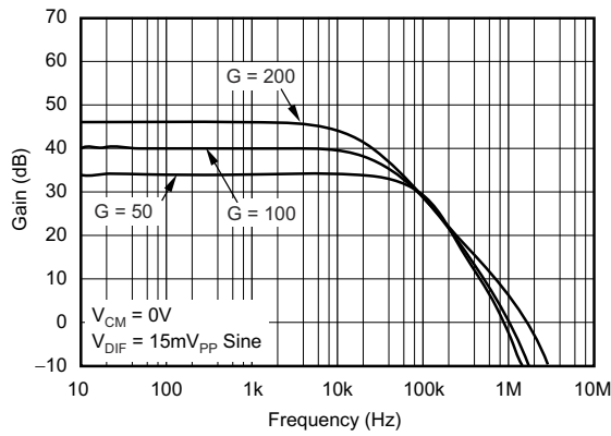
图 6-3. 增益与频率的关系
