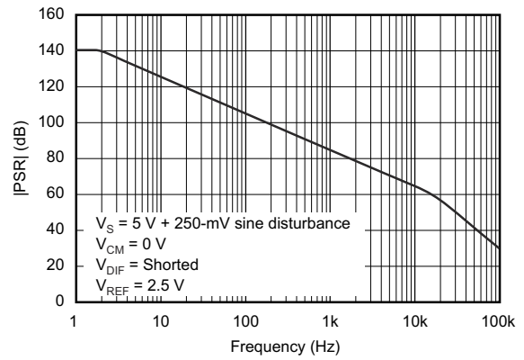
图 6-4. 电源抑制比与频率之间的关系
