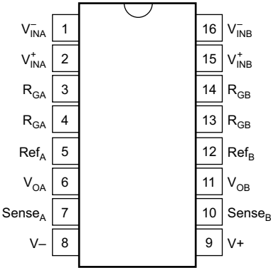
图 4-2. INA2126 : N ( 16 引脚 PDIP ) 、 D ( 16 引脚 SOIC ) 以及 DBQ ( 16 引脚 SSOP ) 封装，顶视图
