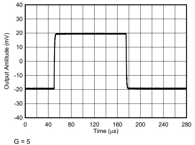
图 5-18. 小信号响应
