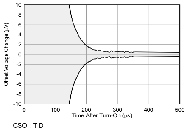
图 5-12. 输入失调电压预热
