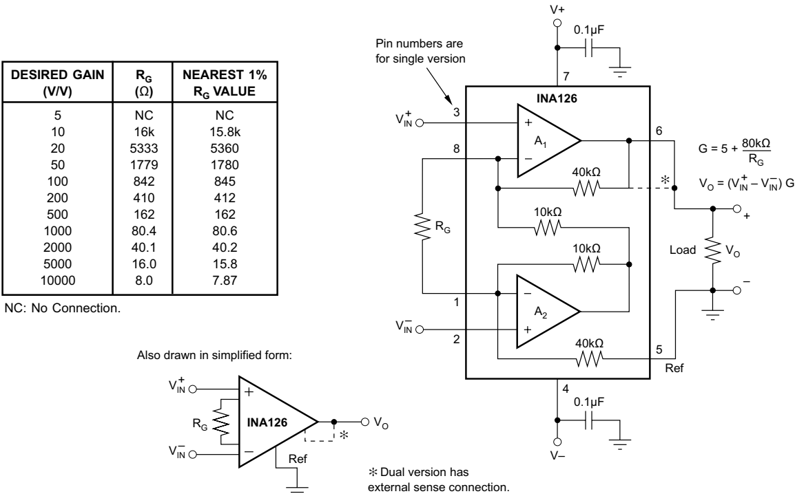
图 7-1. 基本连接
