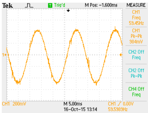
图 7-4. INA126 输入处的共模信号
