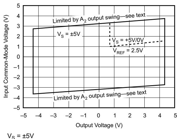
图 5-7. 输入共模电压范围与输出电压间的关系
