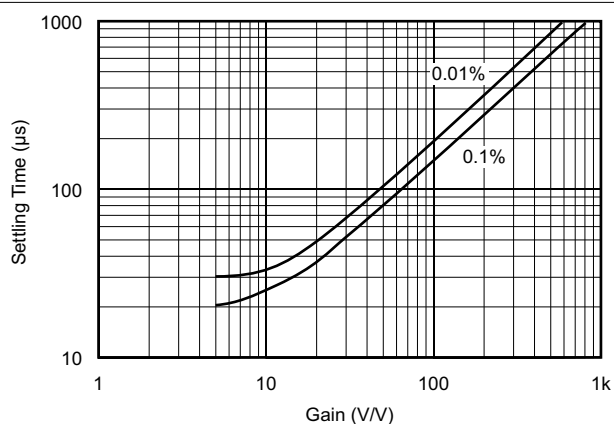
图 5-10. 稳定时间与增益间的关系
