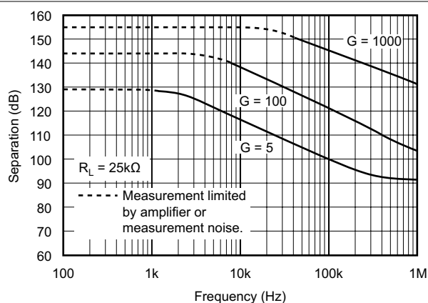
图 5-22. 通道分离与频率间的关系，RTI (双通道版本)
