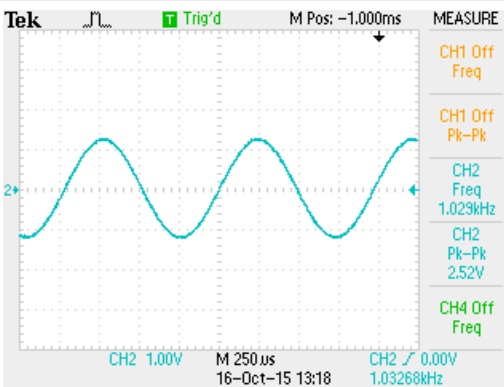
图 7-6. INA126 输出端处的恢复差分信号 (增益为 250)
