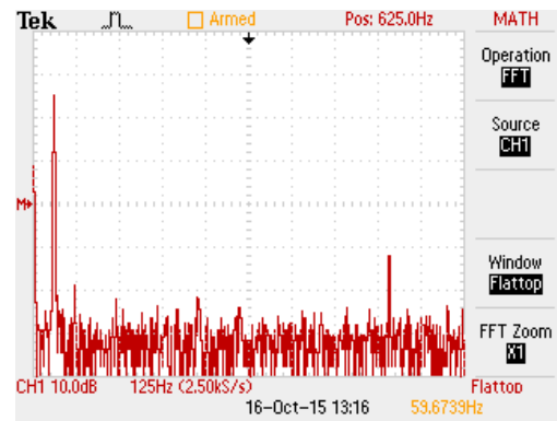
图 7-5. 上图中的信号 FFT 显示了 60Hz 共模及 5kHz 差分信号
