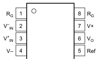
图 4-1. INA126 : P ( 8 引脚 PDIP )、D ( 8 引脚 SOIC ) 以及 DGK ( 8 引脚 VSSOP ) 封装，顶视图
