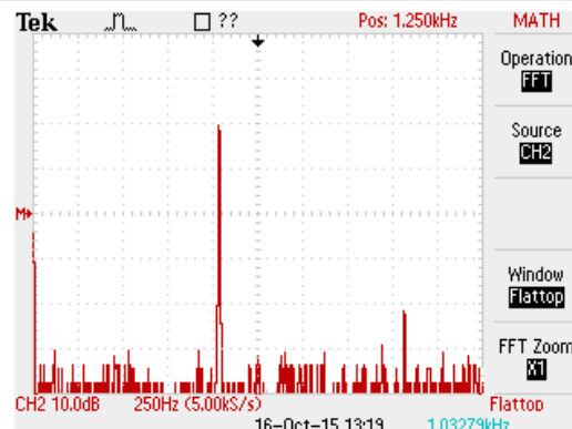
图 7-7. INA126 输出端的 FFT 显示 60Hz 共模信号被抑制
