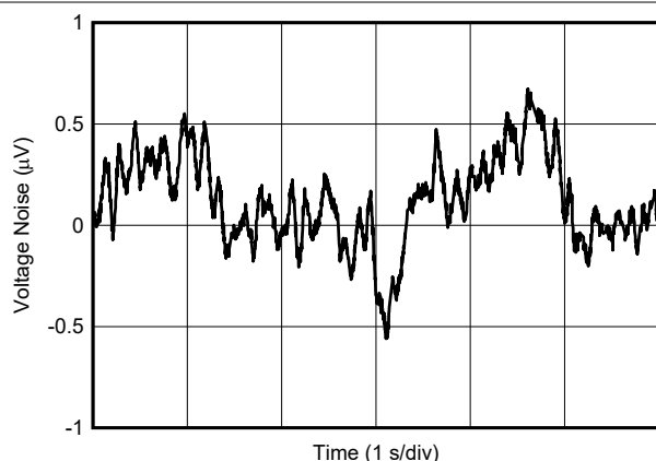
图 5-21. 0.1Hz 至 10Hz 电压噪声
