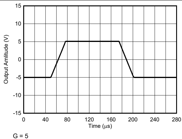
图 5-20. 大信号响应
