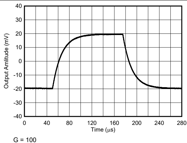
图 5-19. 小信号响应
