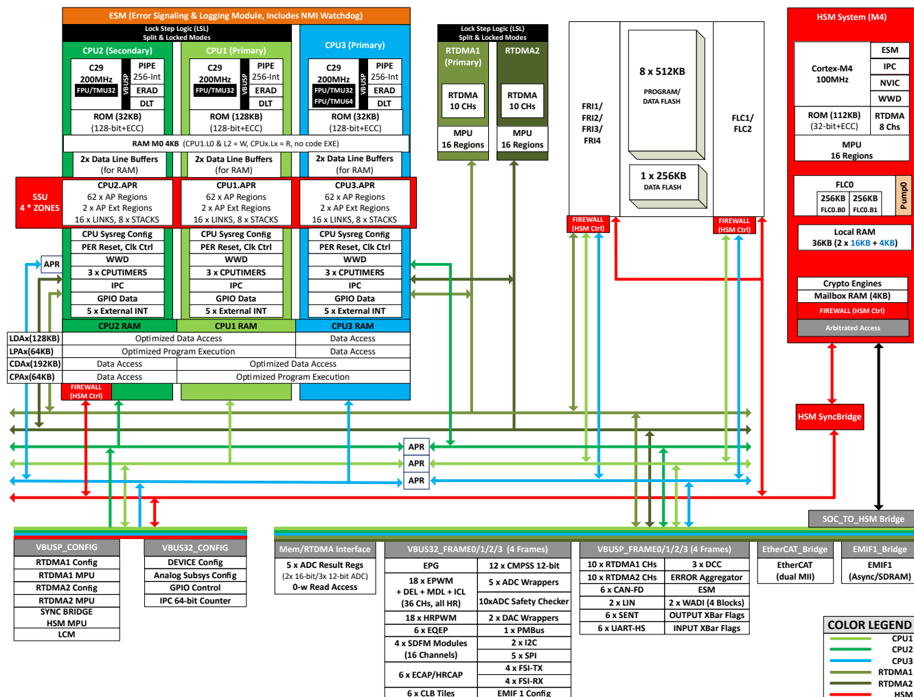
图 3-1. 功能方框图
