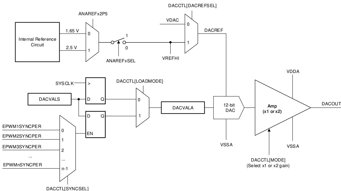
图 6-61. DAC 模块方框图
