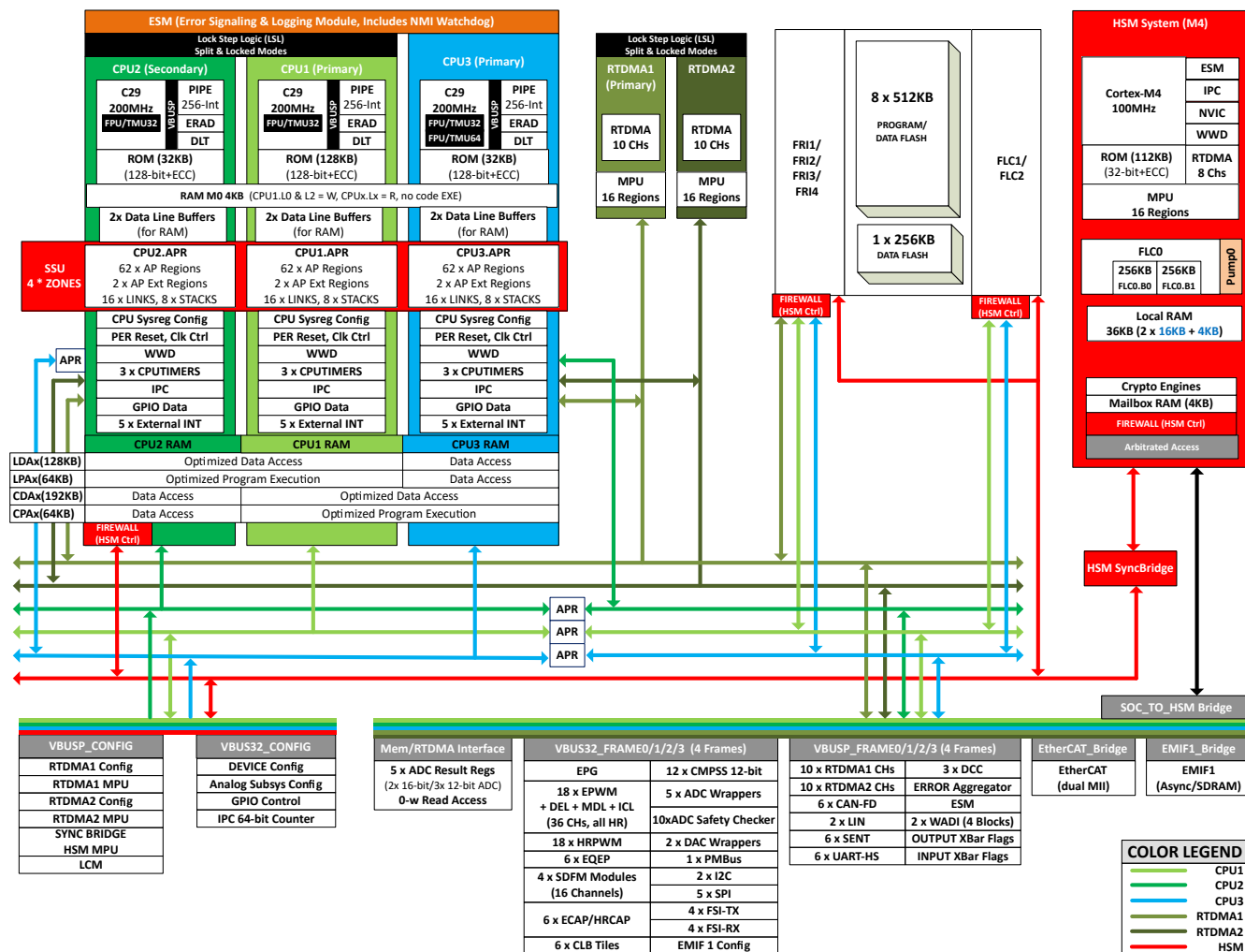
图 7-1. 功能方框图
