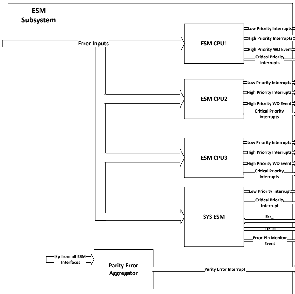
图 7-3. ESM-SS 方框图
