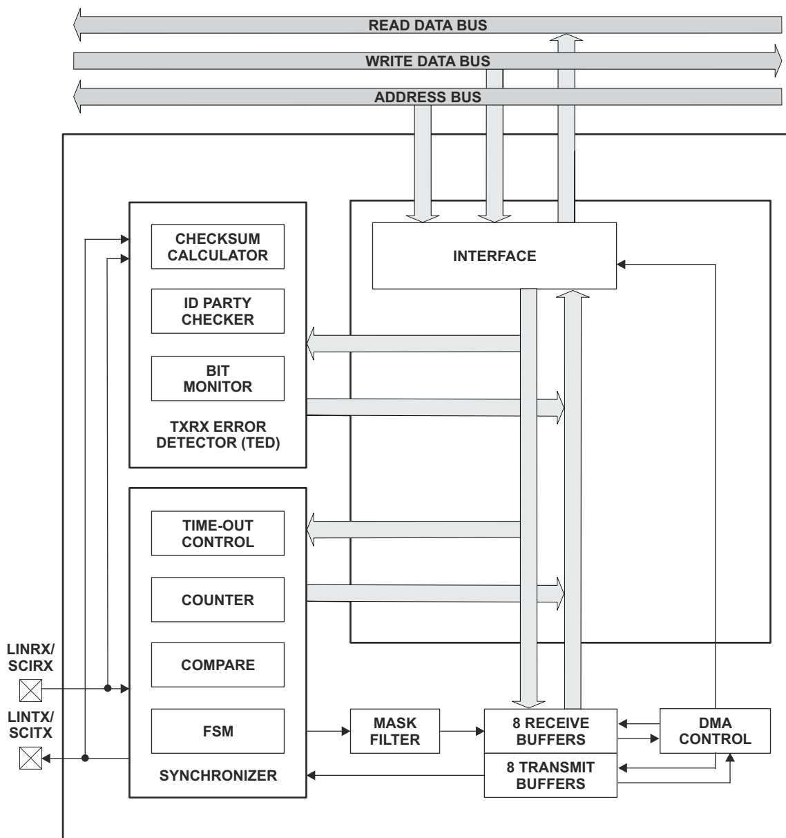
图 6-90. LIN 方框图
