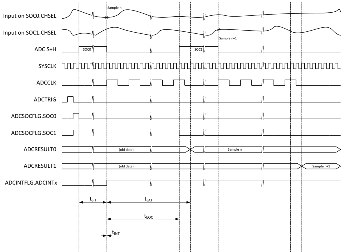
图 6-49. 提前中断模式下 12 位模式的 ADC 时序
