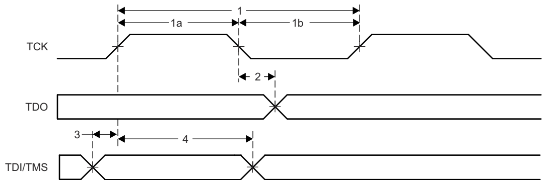
图 6-18. JTAG 时序
