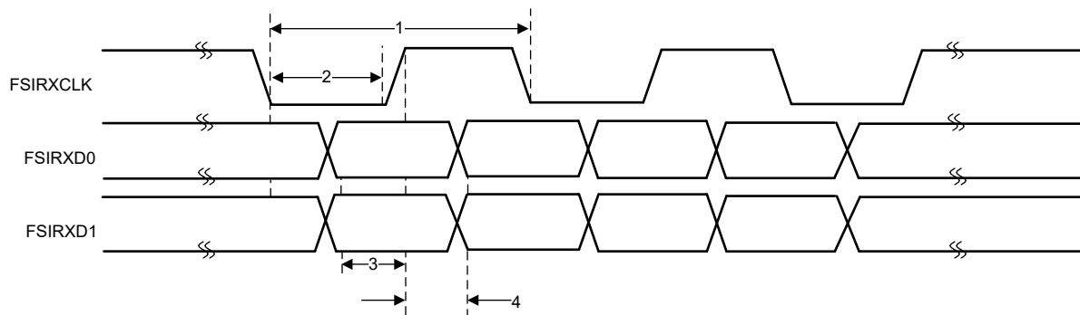
图 6-80. FSIRX 时序
