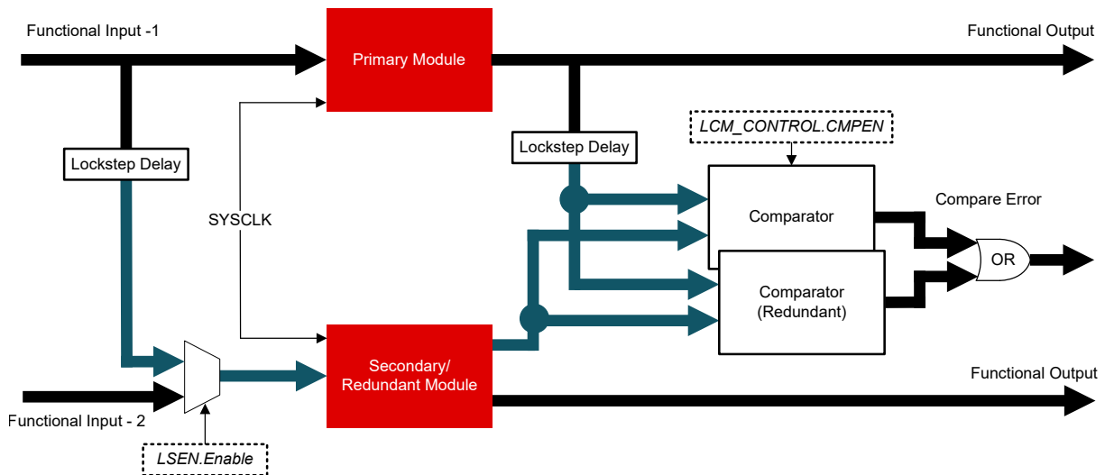
图 7-23. LCM 方框图
