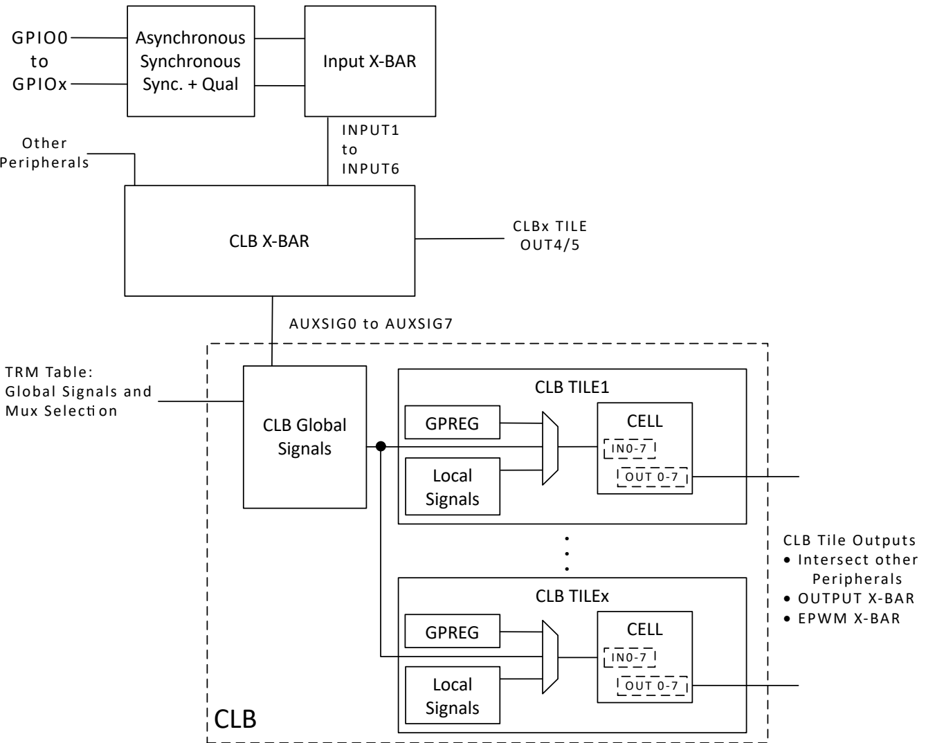
图 7-22. GPIO 到 CLB 逻辑块的连接
