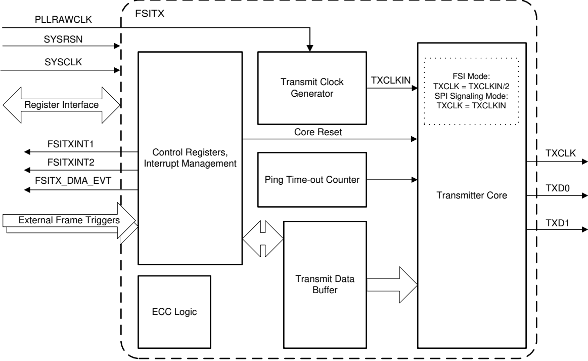
图 6-76. FSITX 方框图
