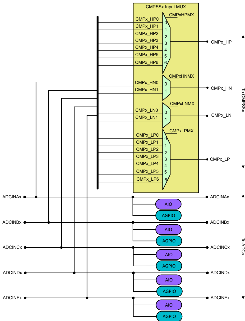
图 6-34. 模拟组连接
