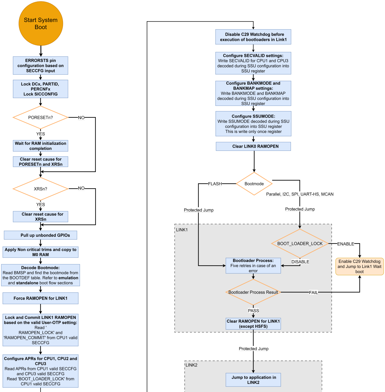
图 7-9. 应用程序代码的系统引导流程
