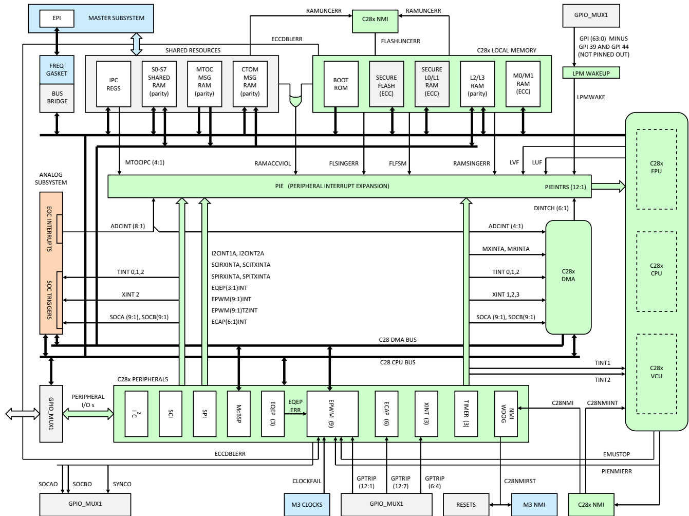
图 8-2. Control Subsystem
