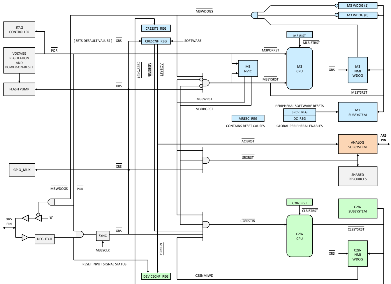
图 8-5. Resets
