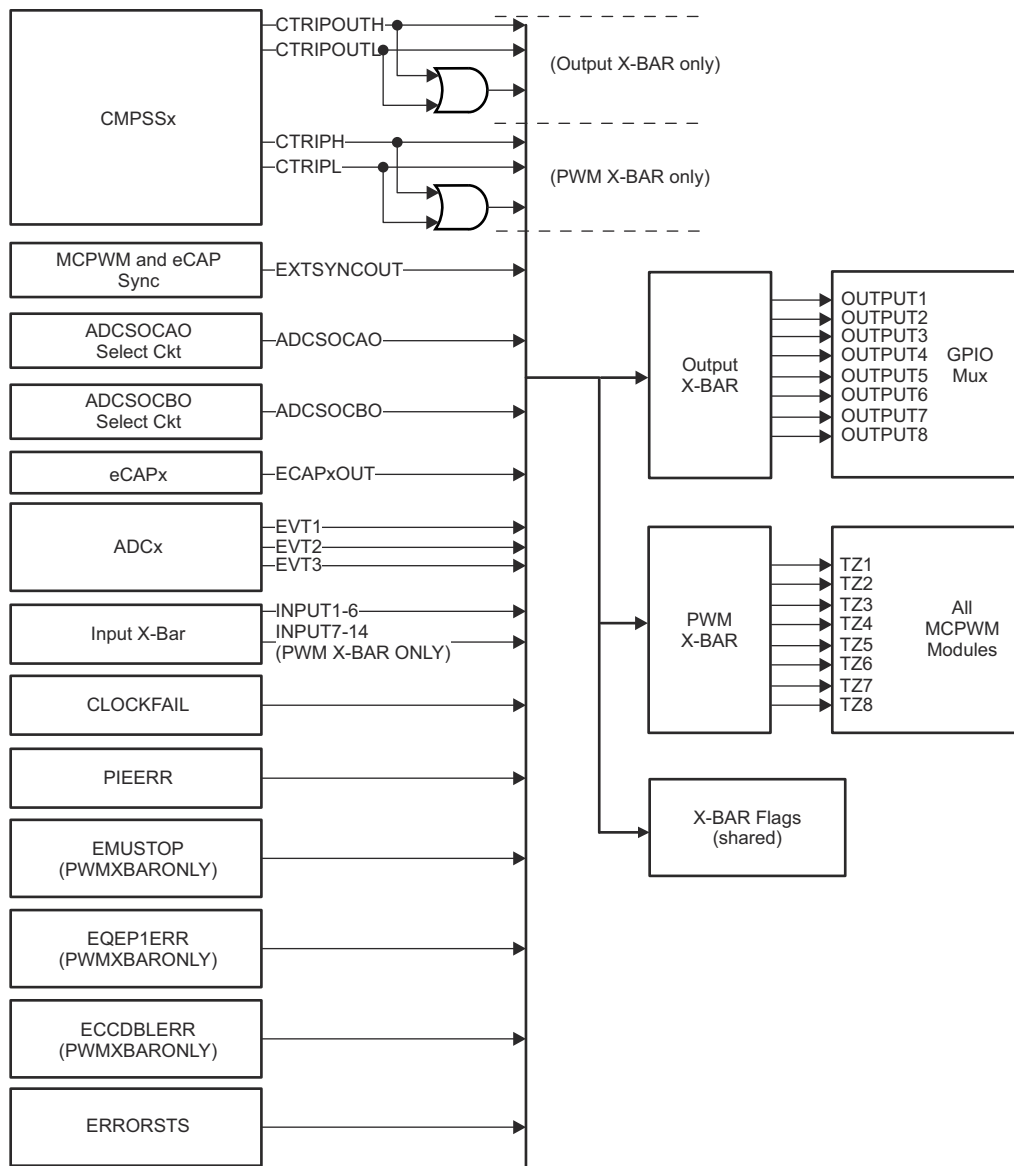
图 5-3. 输出 X-BAR 和 ePWM X-BAR
