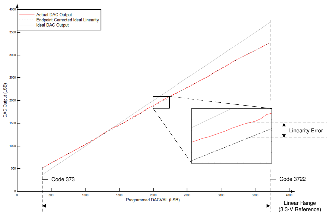
图 6-49. 缓冲 DAC 线性
