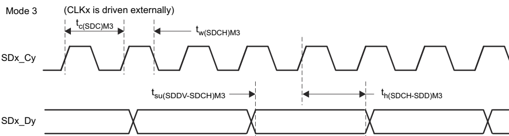
图 6-62. SDFM 时序图 - 模式 3
