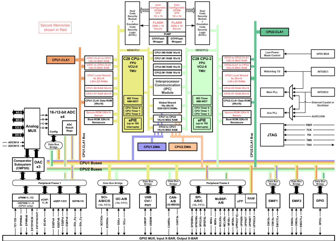
图 3-1. F2837xD 功能框图
