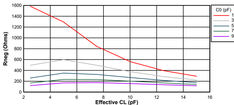
图 6-13. 20MHz 时的负电阻变化
