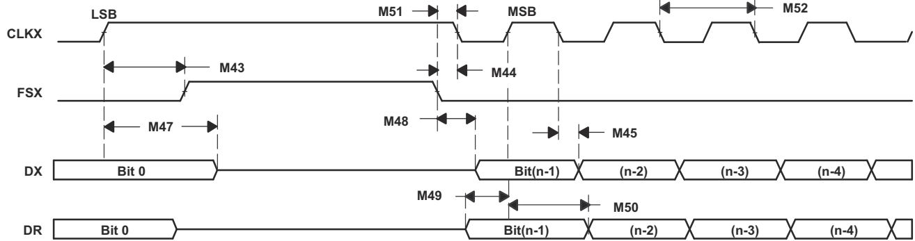
图 6-71. McBSP 时序作为 SPI 主器件或从器件：CLKSTP=10b，CLKXP=1
