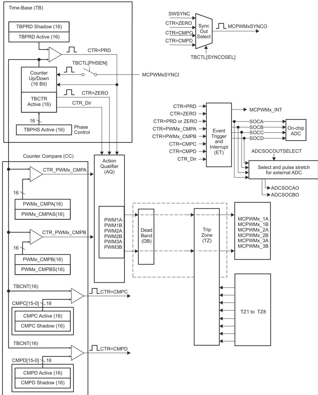
图 6-52. ePWM 子模块和关键内部信号互连
