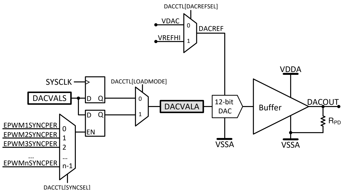
图 6-46. DAC 模块方框图
