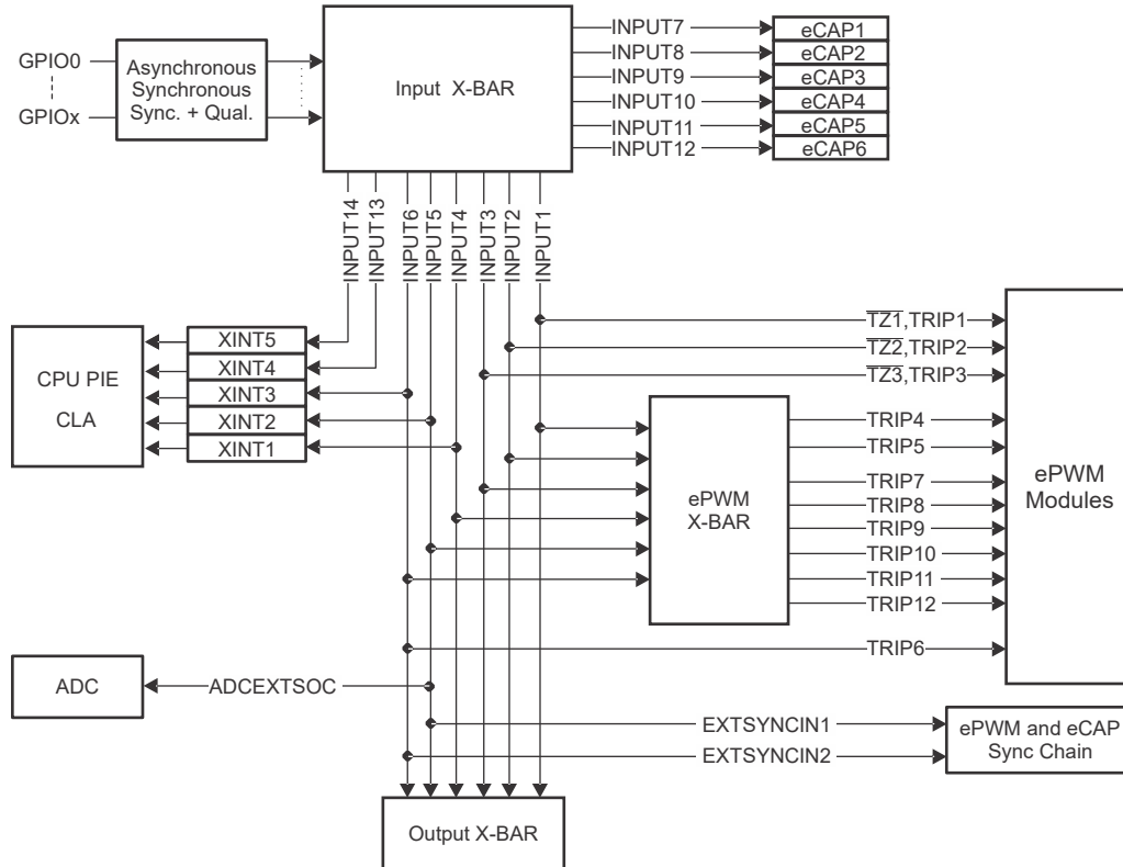
图 5-2. 输入 X-BAR
