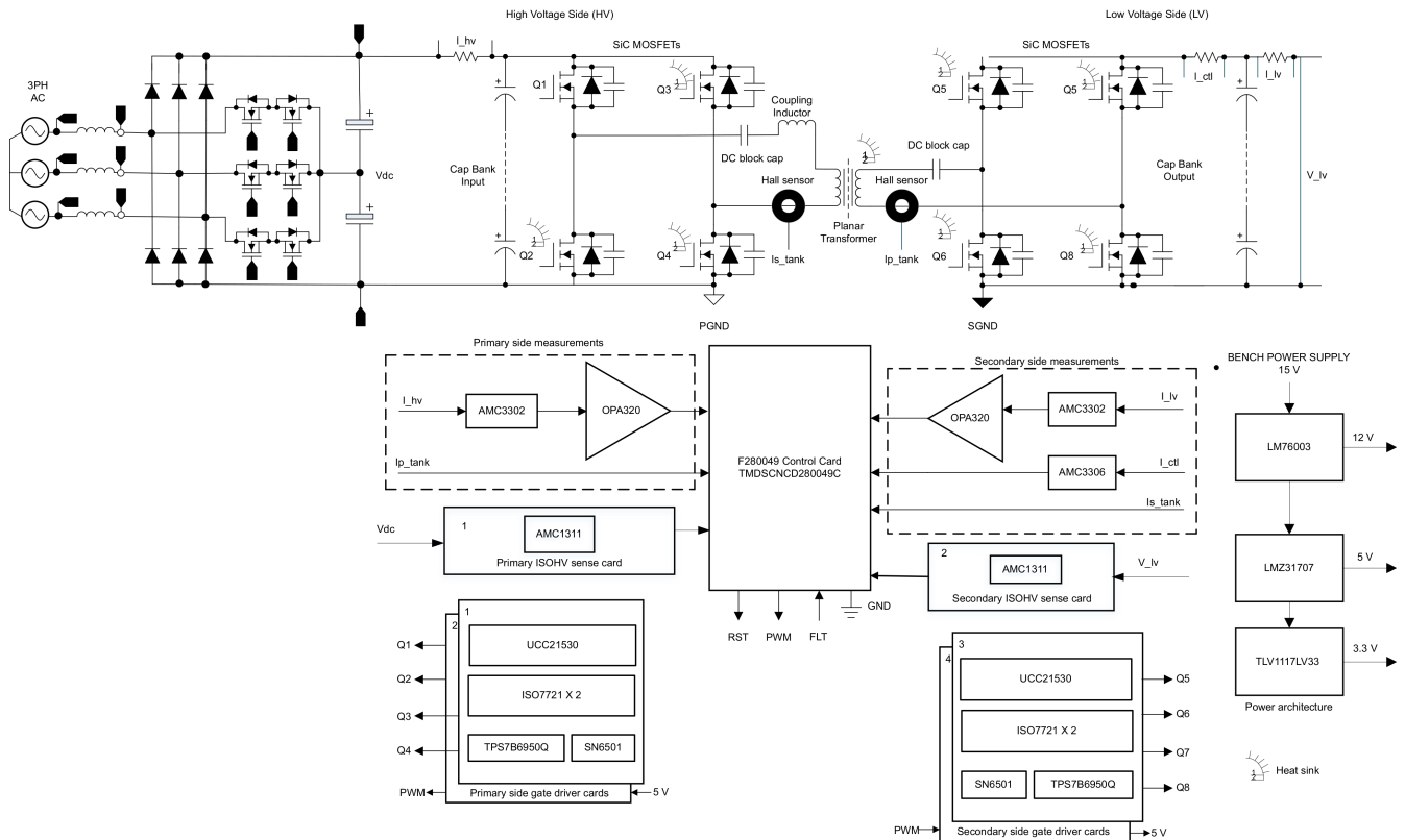
图 8-3. 双有源电桥直流/直流转换器
