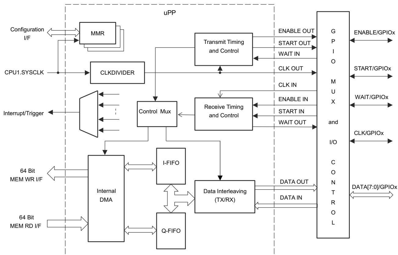
图 6-81. uPP 功能方框图
