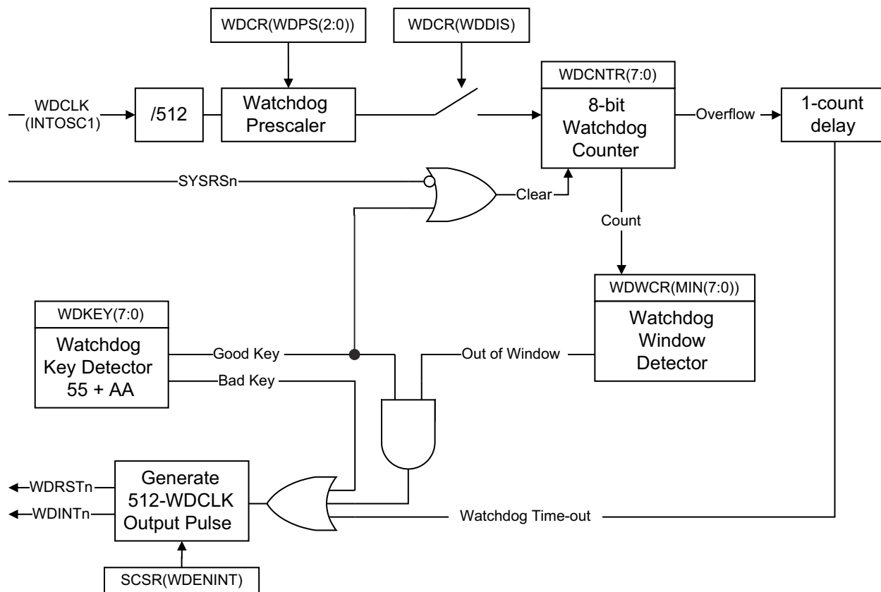
图 7-5. 窗口看门狗
