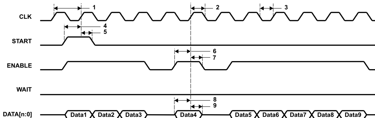
图 6-82. uPP 单倍数据速率 (SDR) 接收时序
