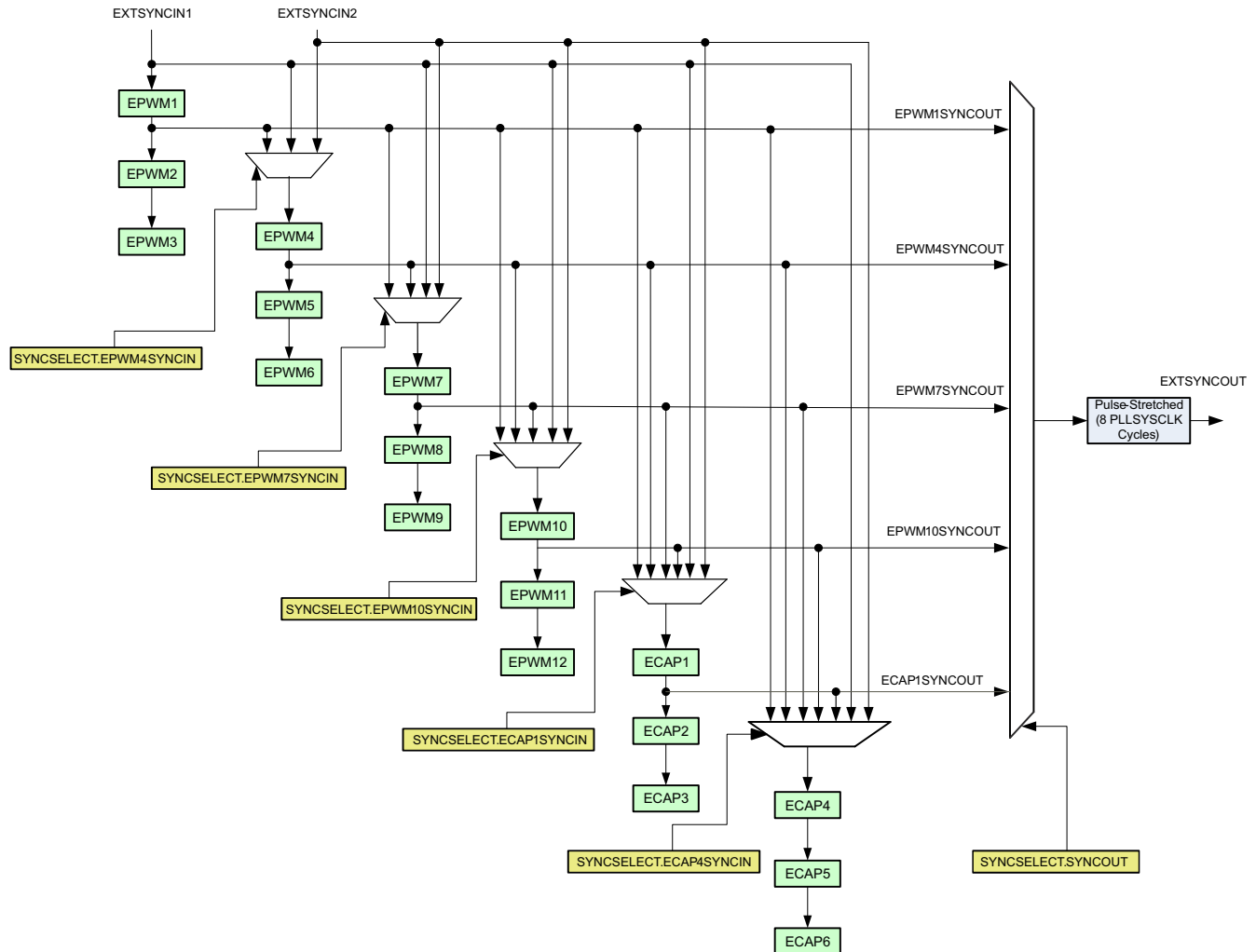
图 6-54. 同步链架构
