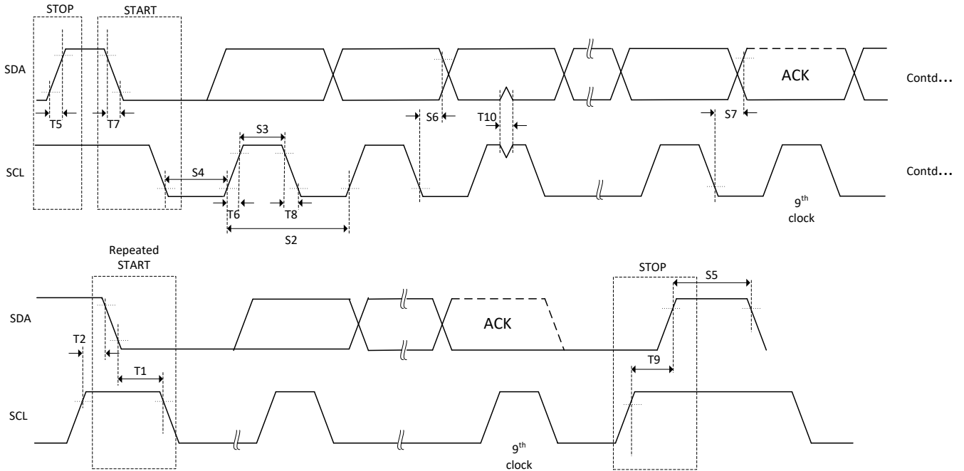
图 6-65. I2C 时序图
