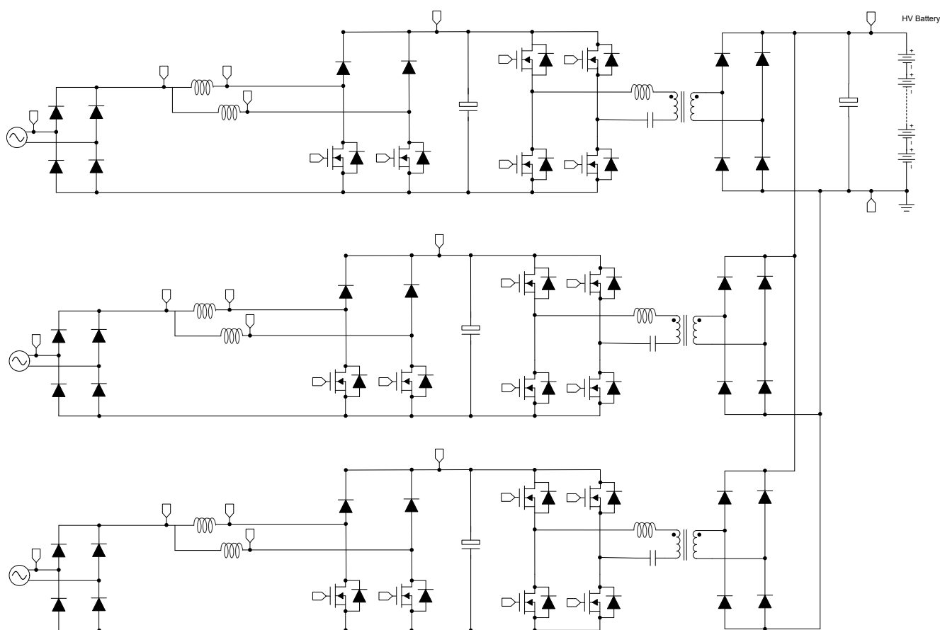
图 8-2. 11kW 模块化 OBC 电源拓扑 (单向、桥式 PFC)
