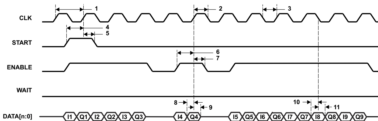
图 6-83. uPP 双倍数据速率 (DDR) 接收时序
