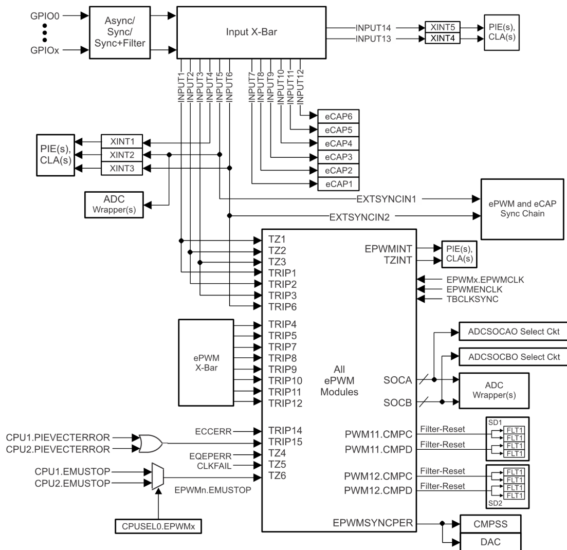
图 6-53. ePWM 跳变输入连接
