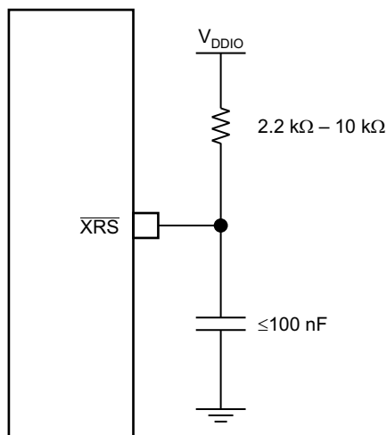
图 6-5. 复位电路
