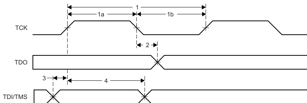
图 6-16. JTAG 时序
