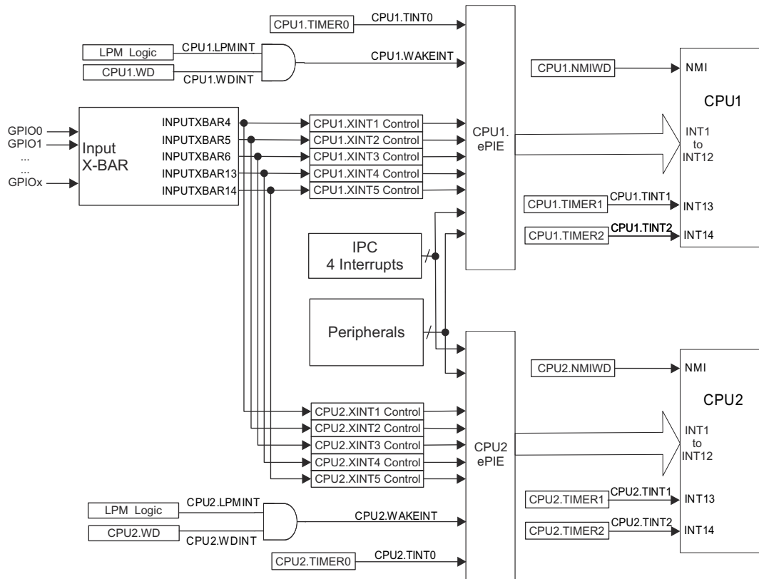
图 6-20. 外部和 ePIE 中断源
