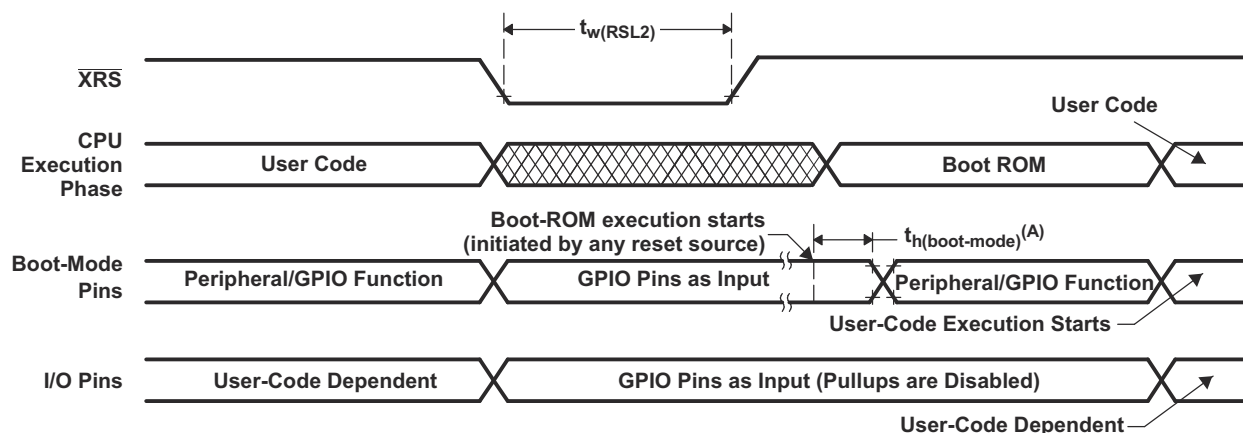
图 6-6. 上电复位
