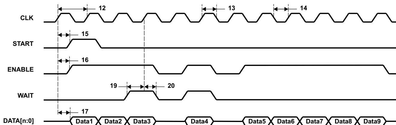
图 6-84. uPP 单倍数据速率 (SDR) 发送时序
