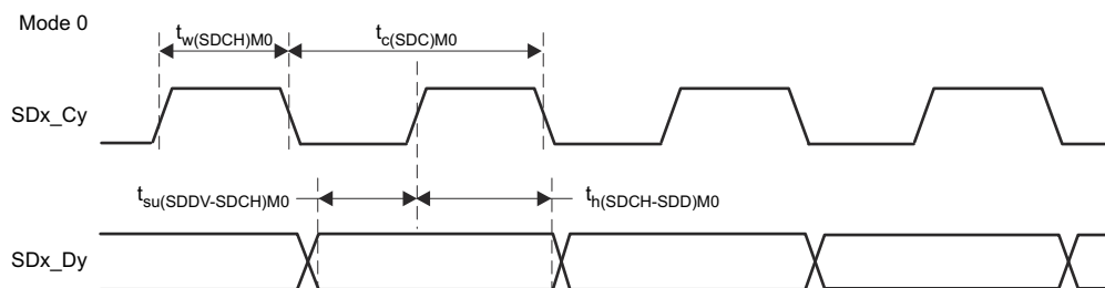
图 6-59. SDFM 时序图 - 模式 0
