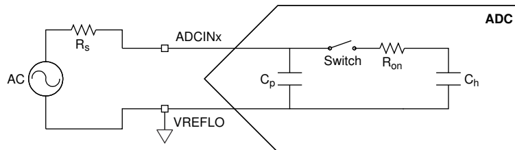
图 6-37. 单端输入模型
