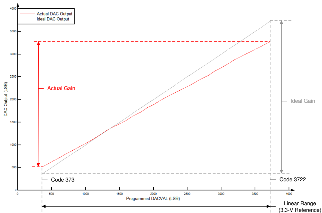
图 6-48. 缓冲 DAC 增益
