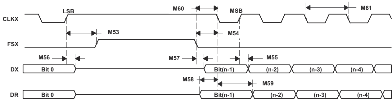
图 6-72. McBSP 时序作为 SPI 主器件或从器件：CLKSTP=11b，CLKXP=1
