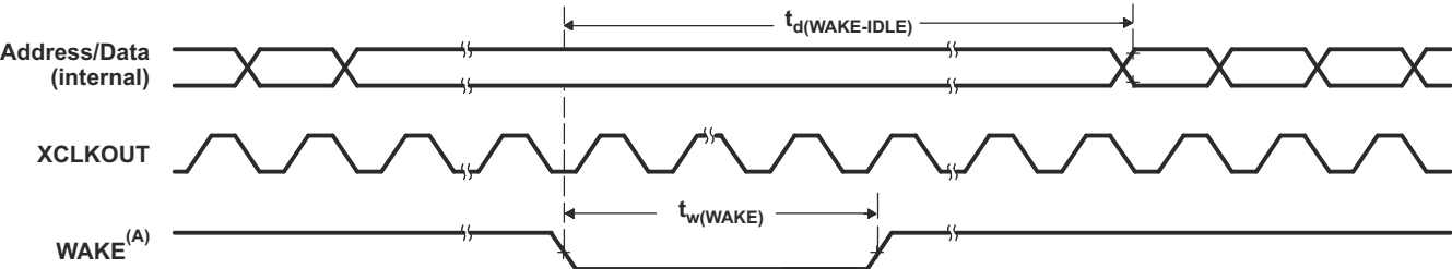
图 6-22. 空闲进入和退出时序图
