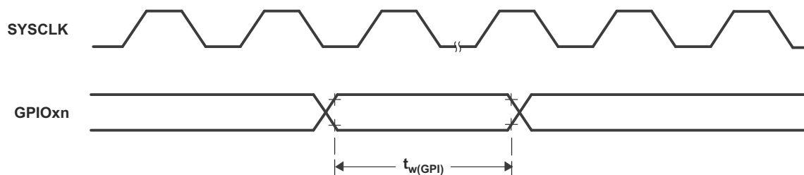
图 6-19. 通用输入时序
