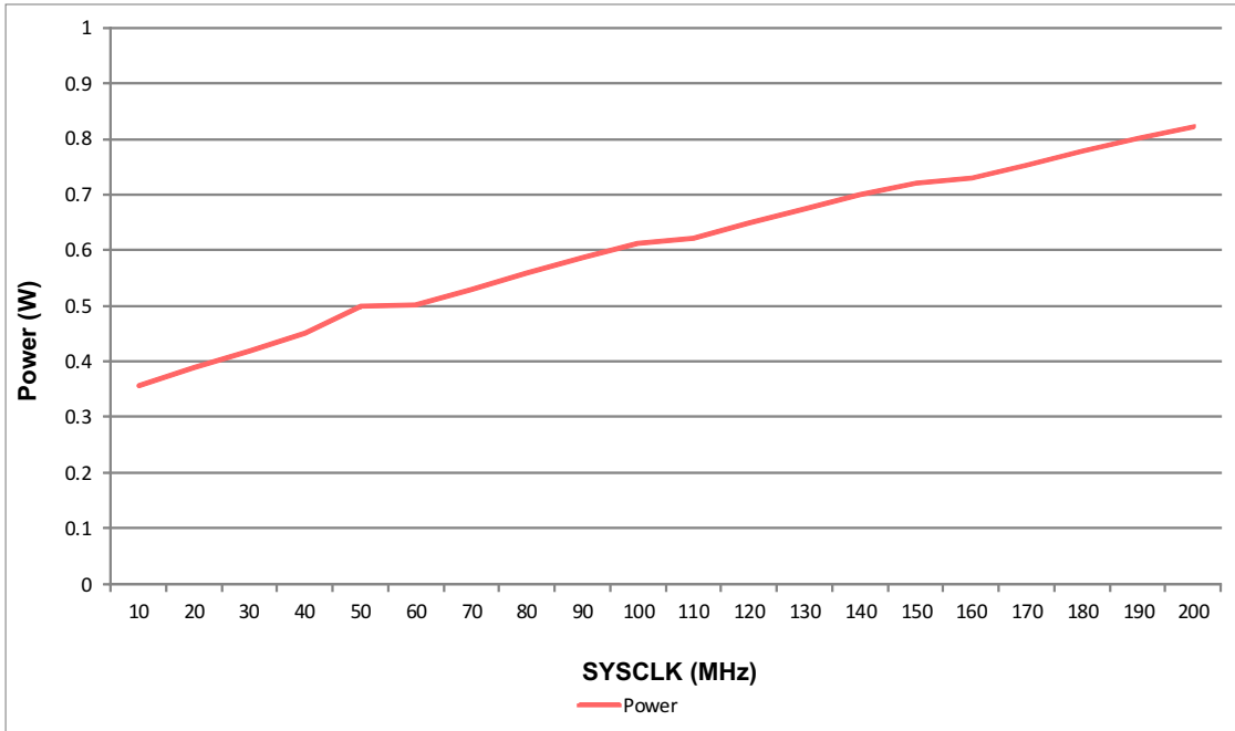
图 6-3. 功率与频率间的关系
