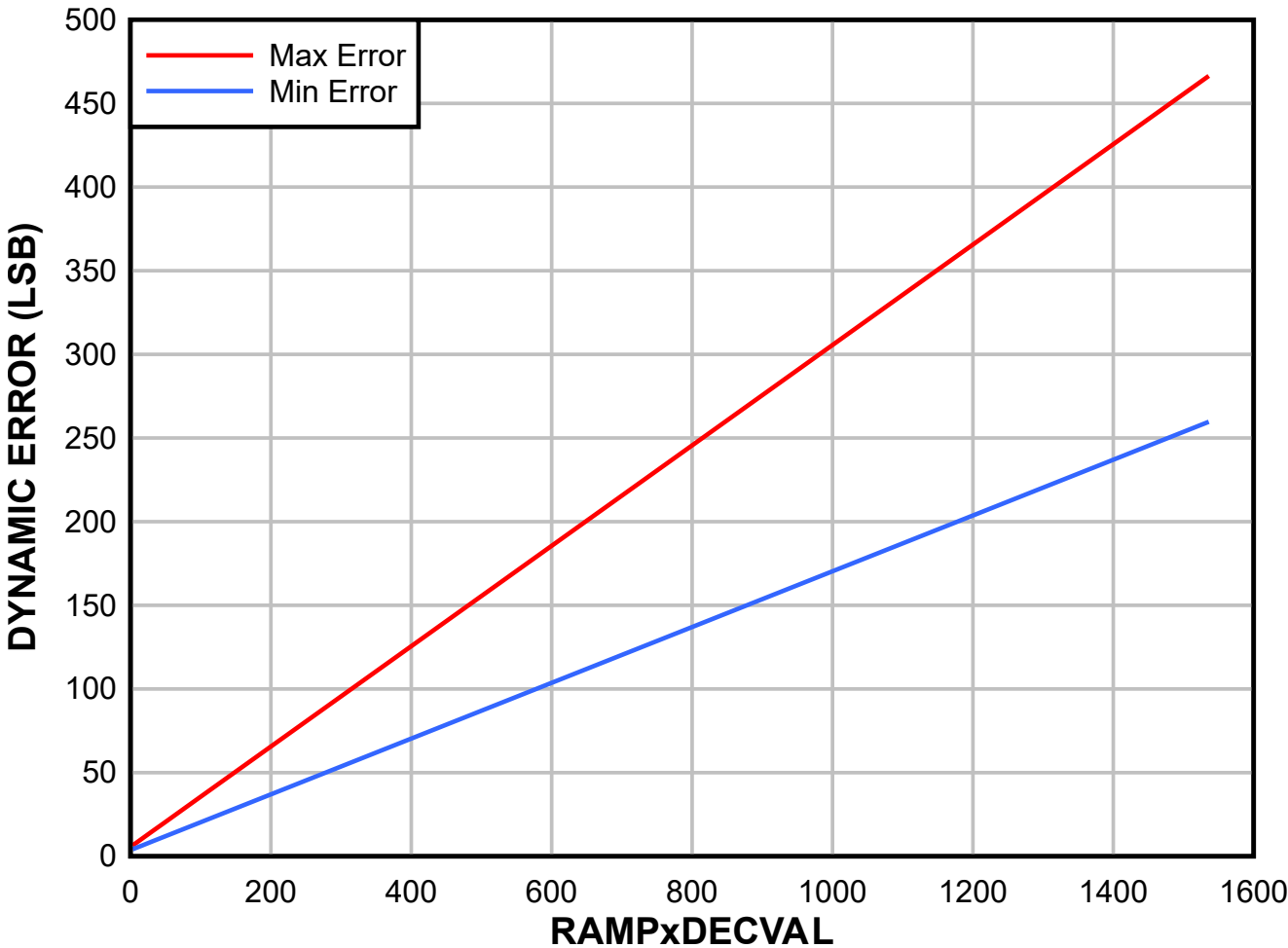
图 6-50. CMPSS DAC 动态误差
