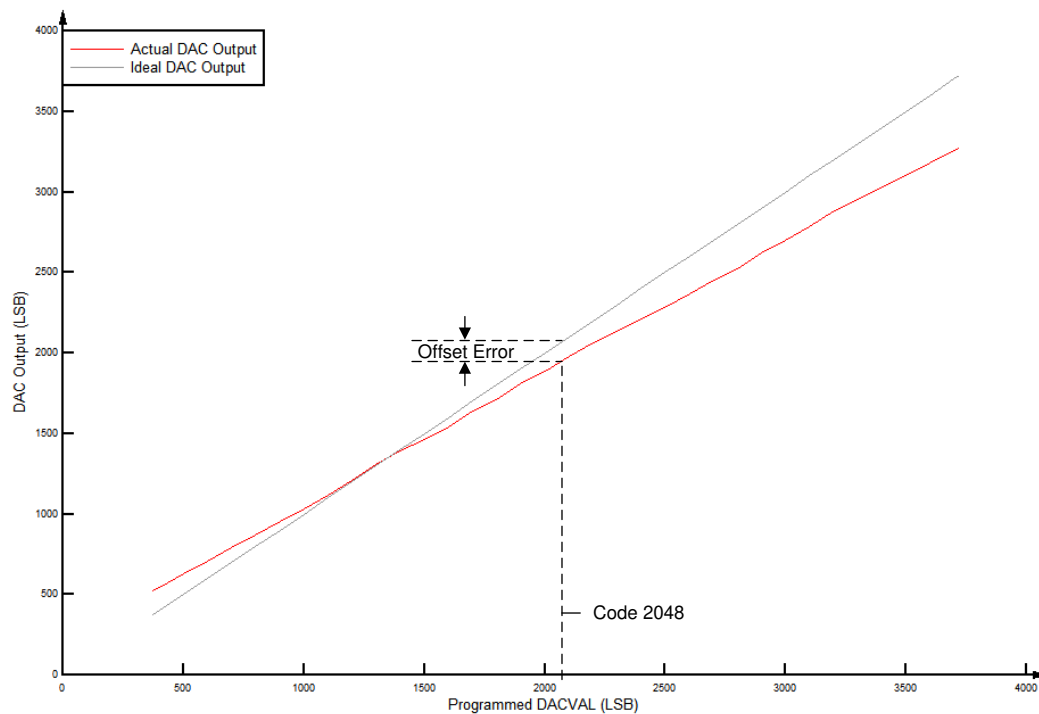
图 6-47. 缓冲 DAC 偏移
