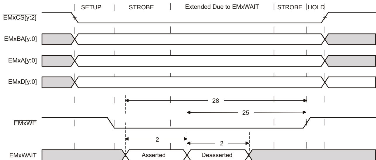
图 6-29. \text{EMxWAIT} 写入时序要求
