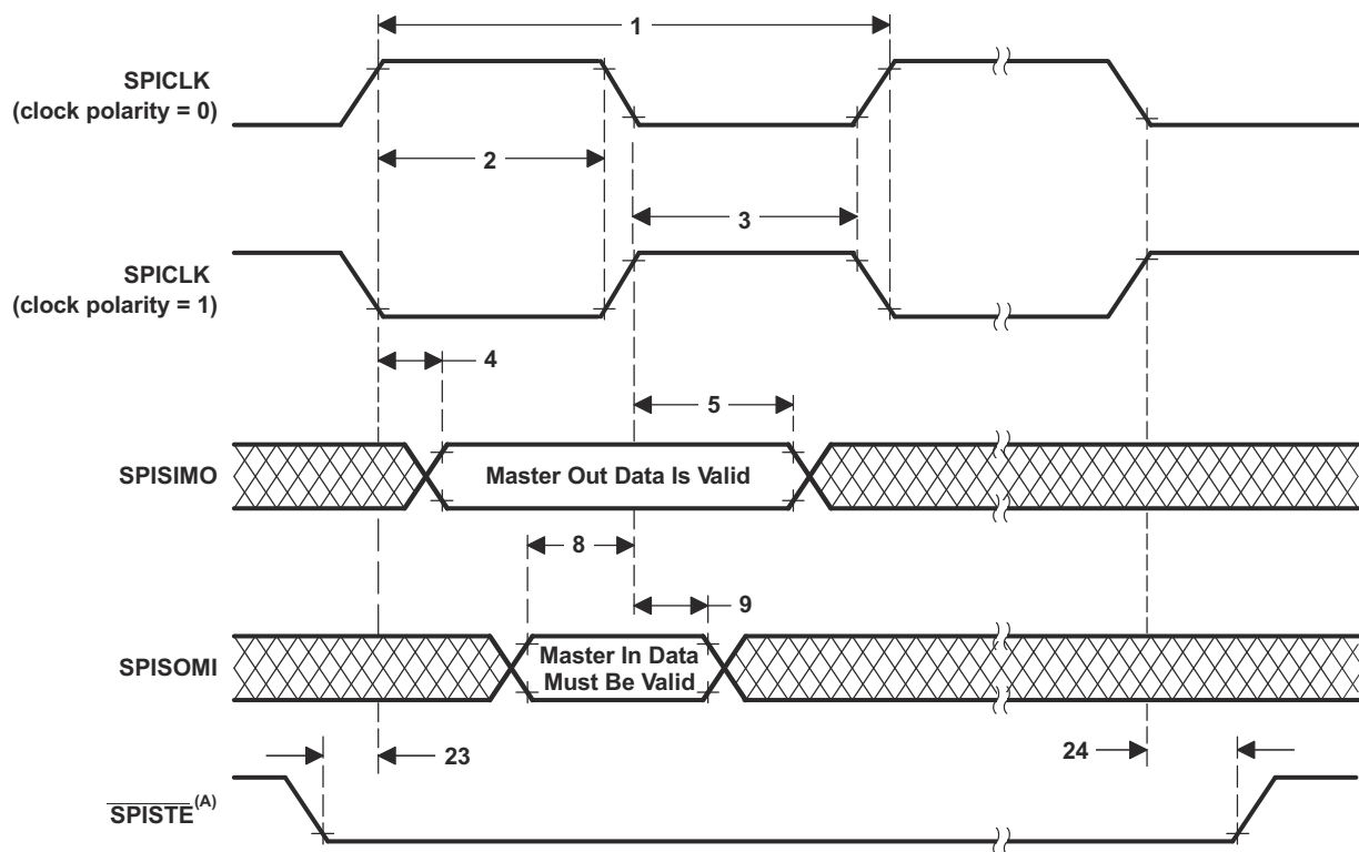
图 6-75. SPI 主模式外部时序 (时钟相位 = 0)
