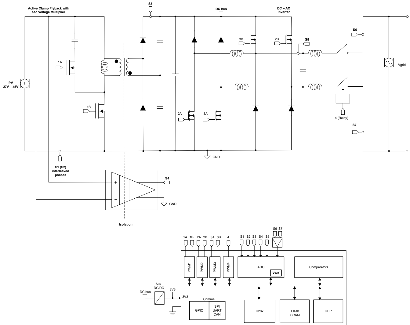
图 8-1. 微型光伏逆变器
