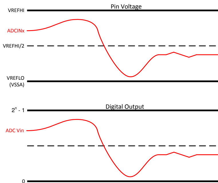
图 6-35. 单端信号模式
