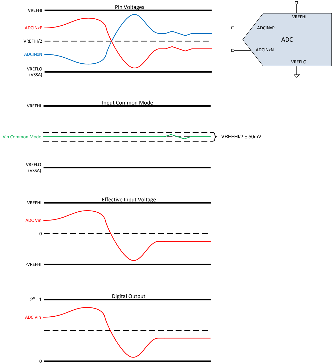
图 6-34. 差分信号模式
