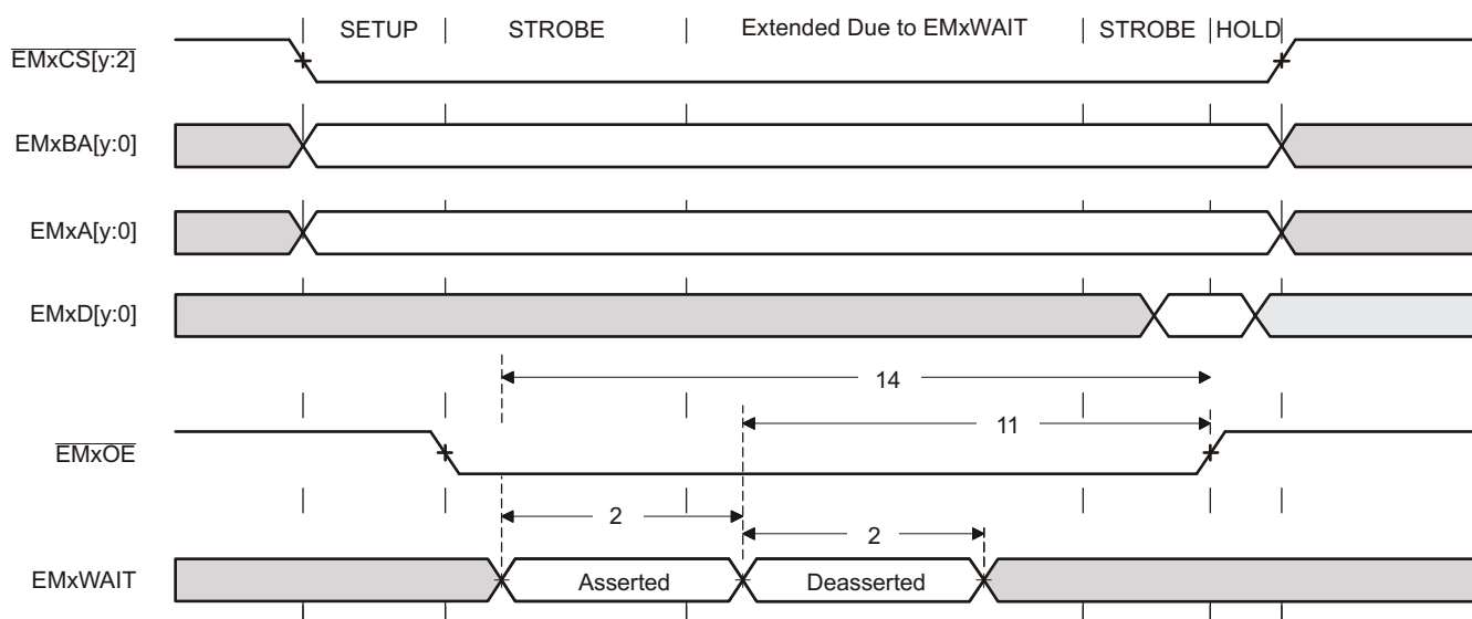
图 6-27. EMxWAIT 读取时序要求
