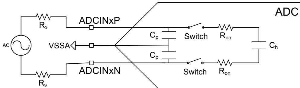
图 6-36. 差分输入模型
