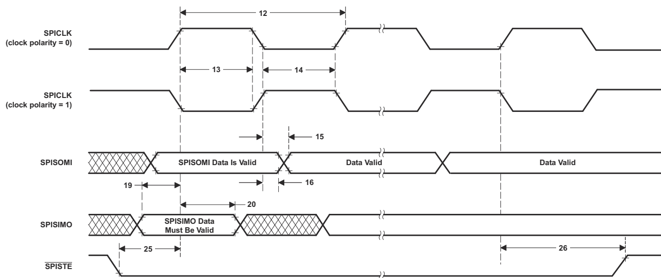
图 6-78. SPI 从模式外部时序 ( 时钟相位 = 1 )
