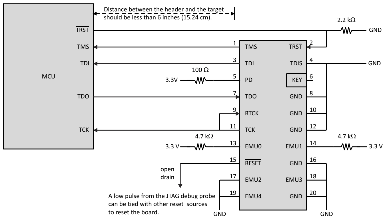
图 6-15. 连接到 20 引脚 JTAG 接头
