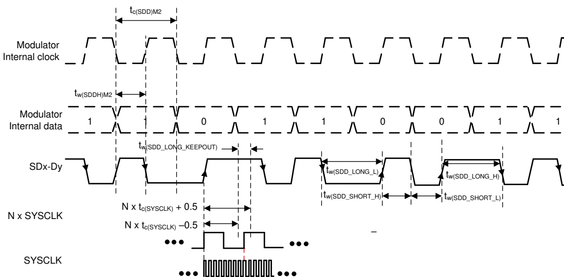
图 6-61. SDFM 时序图 - 模式 2
