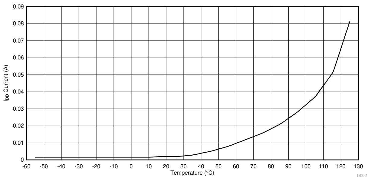
图 6-4. I_{DD} 漏电流与温度间的关系
