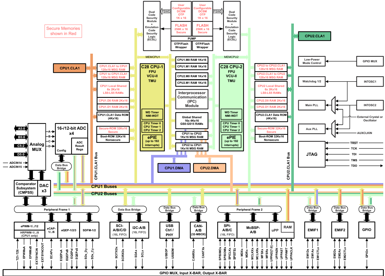
图 7-1. F2837xD 功能框图
