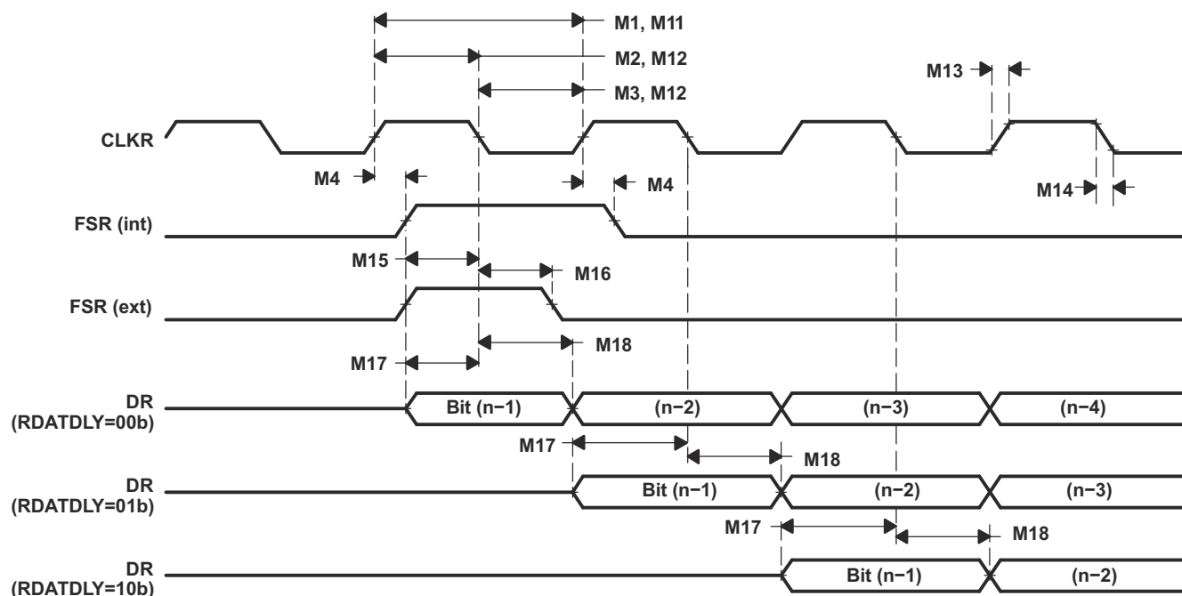
图 6-67. McBSP 接收时序
