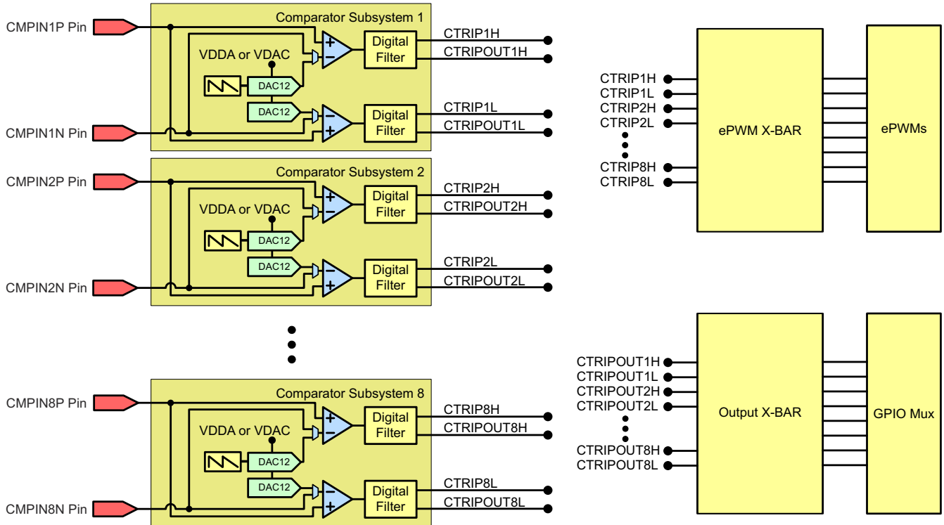
图 6-40. CMPSS 连接 ( 176 引脚 PTP )
