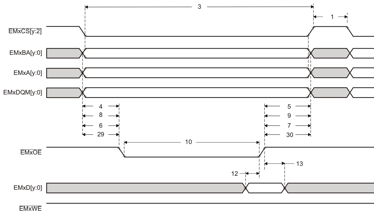
图 6-26. 异步存储器读取时序
