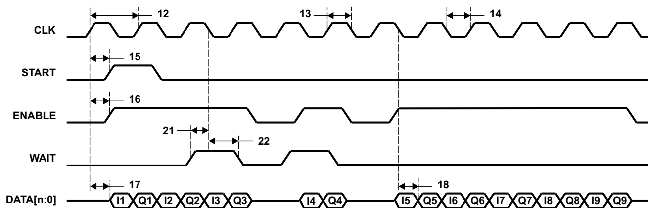
图 6-85. uPP 双倍数据速率 (DDR) 发送时序
