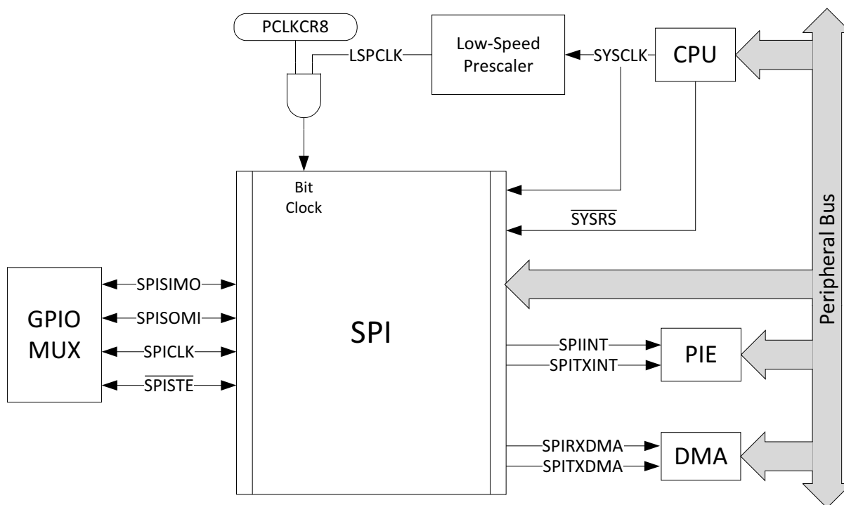
图 6-74. SPI CPU 接口
