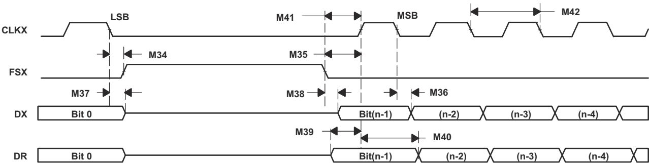
图 6-70. McBSP 时序作为 SPI 主器件或从器件：CLKSTP=11b，CLKXP=0
