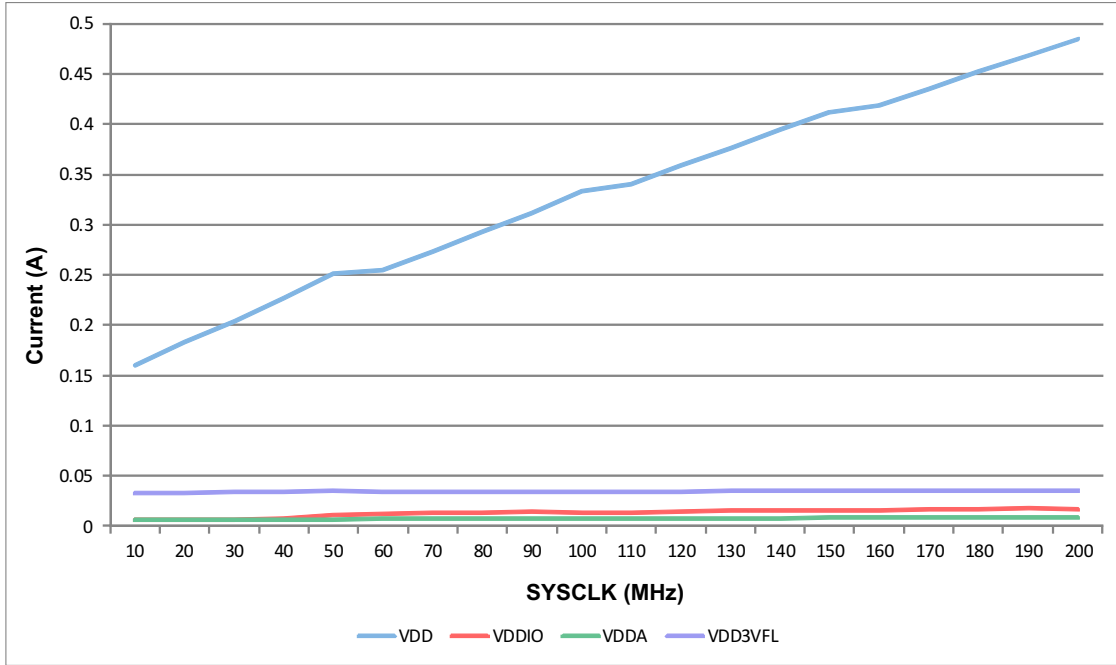
图 6-2. 工作电流与频率间的关系
