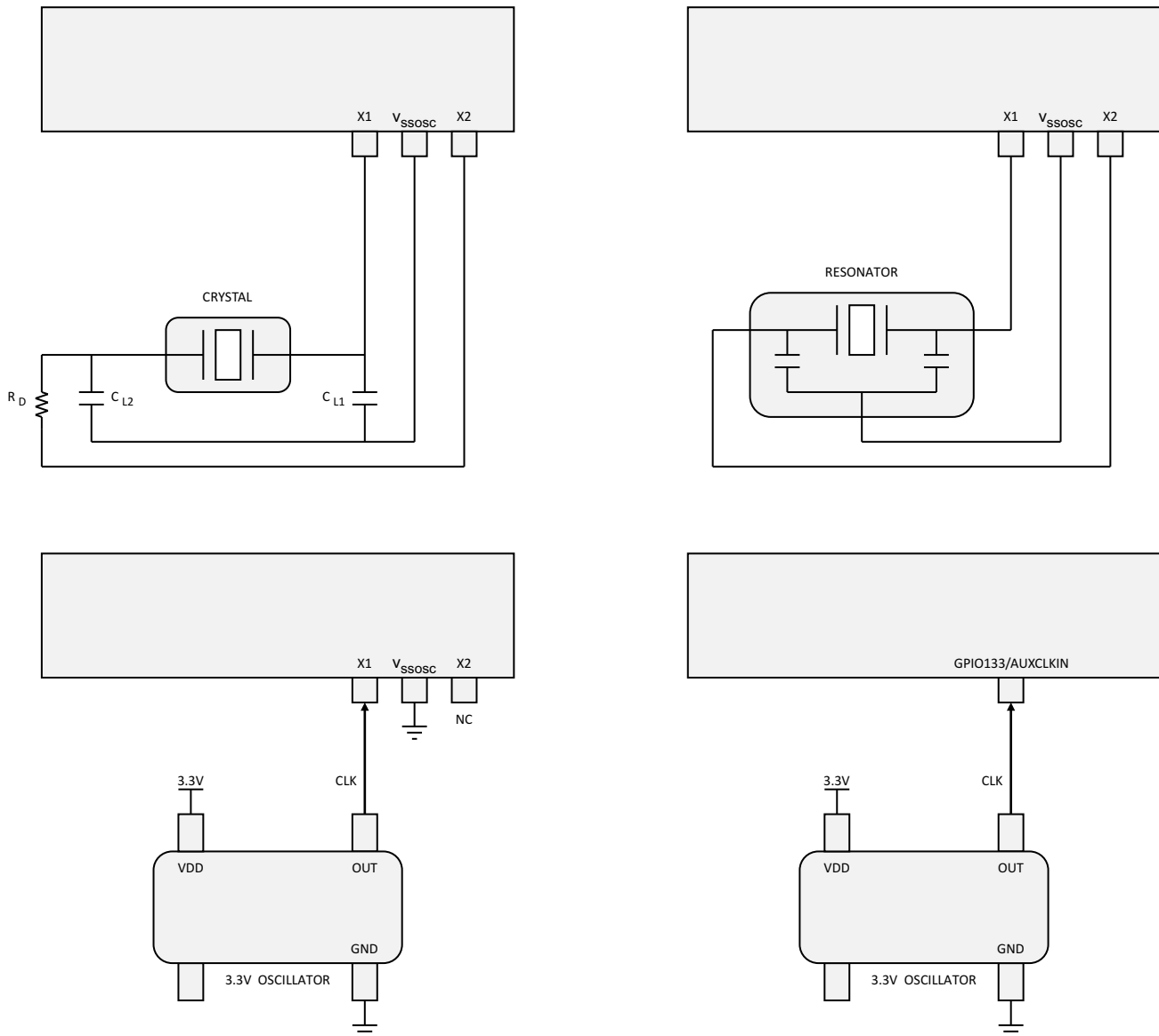
图 6-9. 将输入时钟连接到 F28377D-SEP 器件
