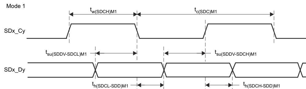
图 6-60. SDFM 时序图 - 模式 1
