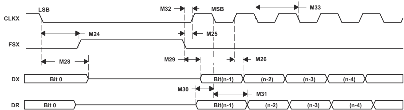
图 6-69. McBSP 时序作为 SPI 主器件或从器件：CLKSTP=10b，CLKXP=0
