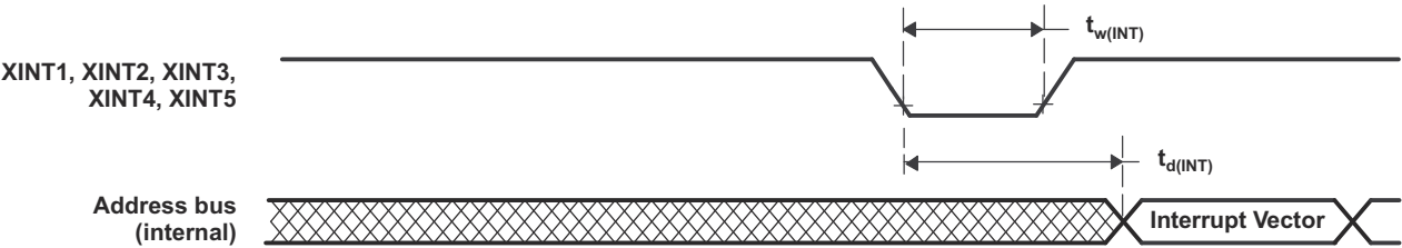
图 6-21. 外部中断时序
