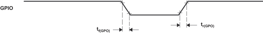
图 6-17. 通用输出时序
