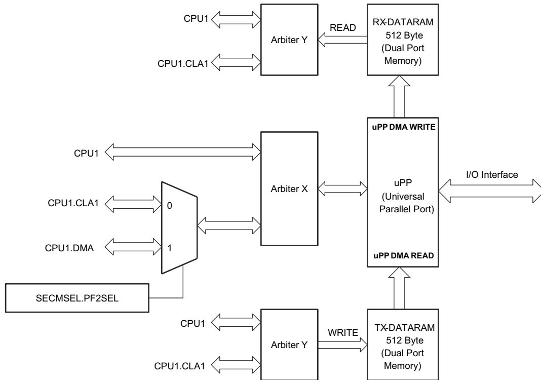
图 6-80. uPP 集成
