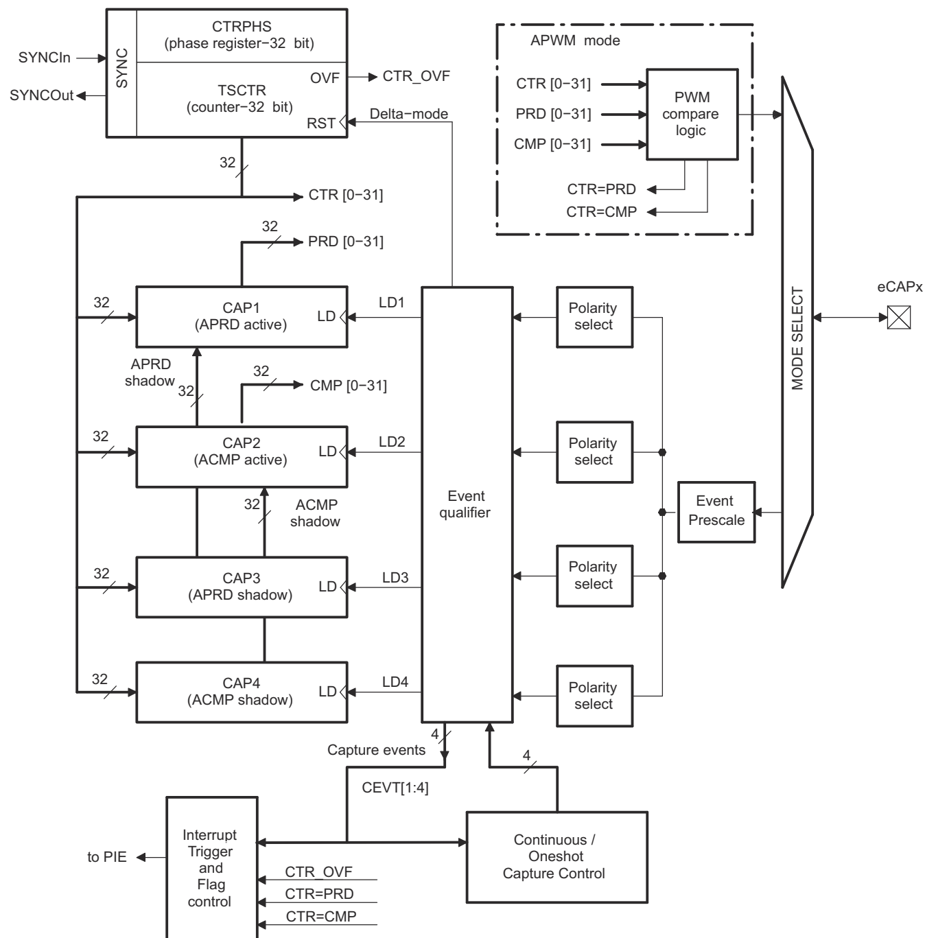
图 6-51. eCAP 方框图
