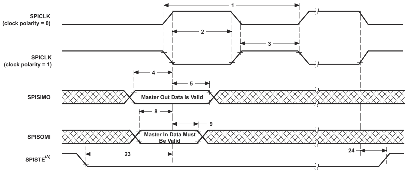
图 6-76. SPI 主模式外部时序 ( 时钟相位 = 1 )
