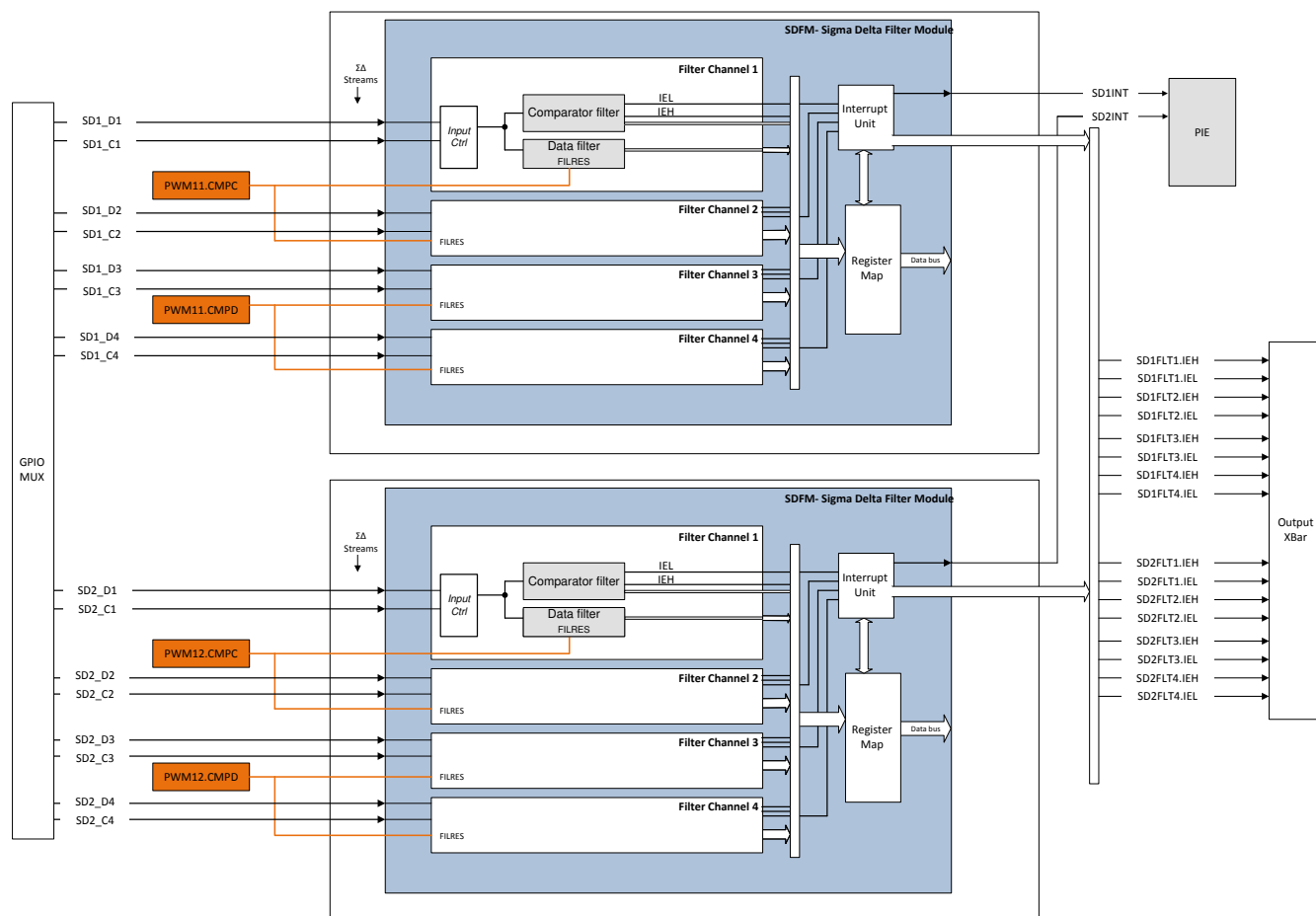
图 6-58. SDFM 方框图
