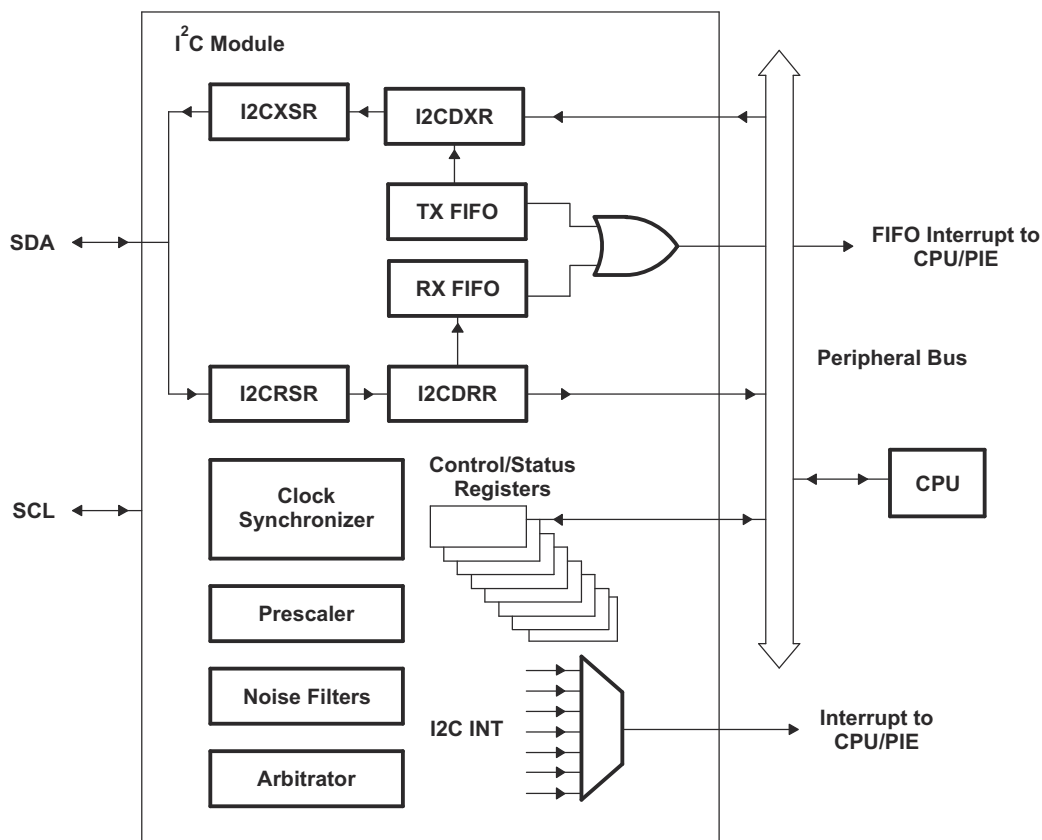
图 6-64. I2C 外设模块接口
