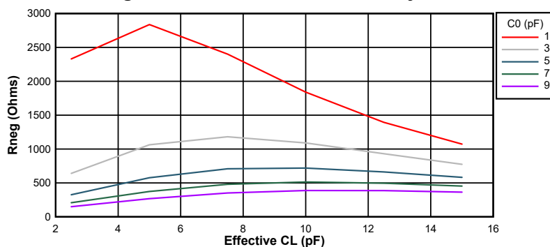
图 6-12. 10MHz 时的负电阻变化
