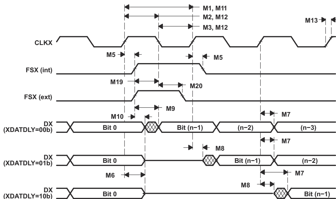
图 6-68. McBSP 传输时序
