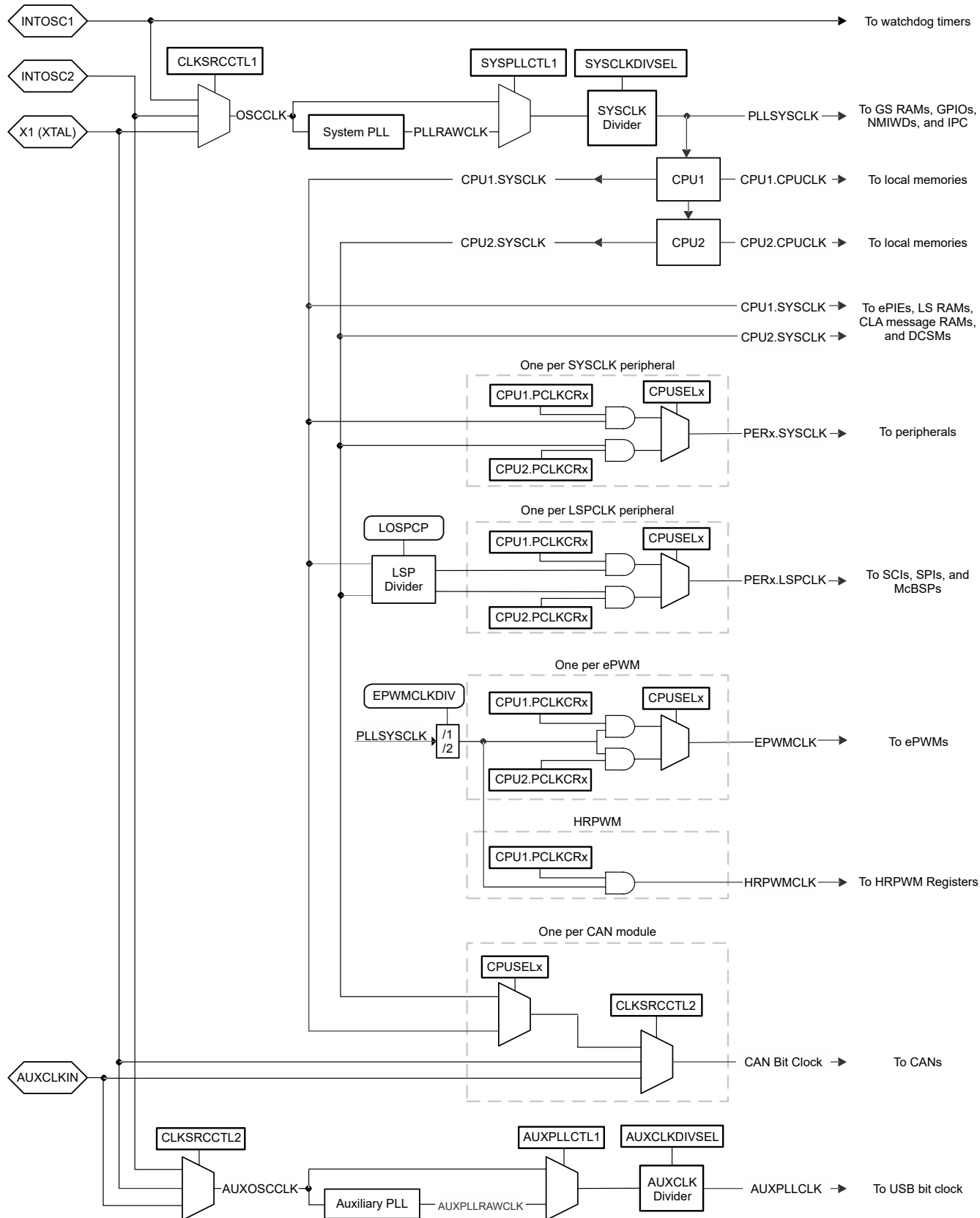
图 6-8. 计时系统
