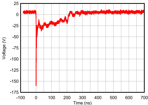
图 7-3. -8kV 钳位 IEC 波形
