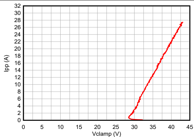
图 5-2. 负 TLP 曲线
