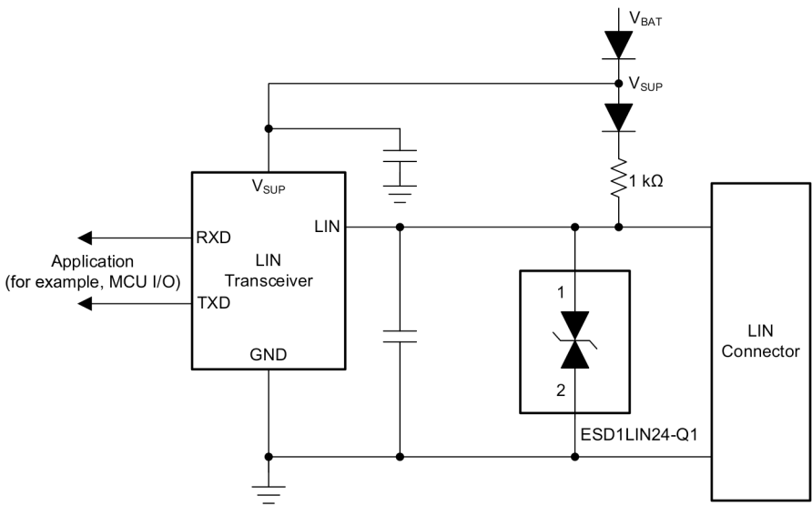
图 7-1. 典型应用
