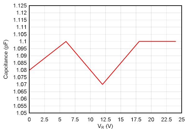
图 5-15. 电容与偏置电压间的关系
