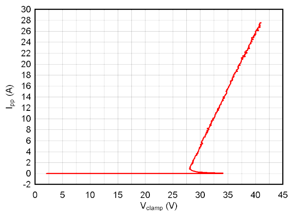
图 5-8. 负 TLP 曲线
