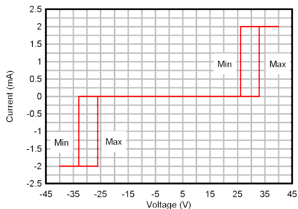
图 5-16. 直流电压扫描 I-V 曲线
