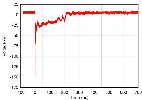
图 5-10. -8kV 钳位 IEC 波形
