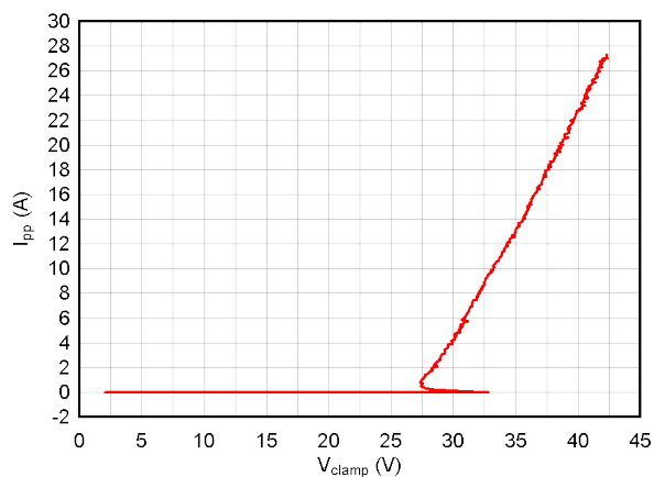
图 5-13. 正 TLP 曲线
