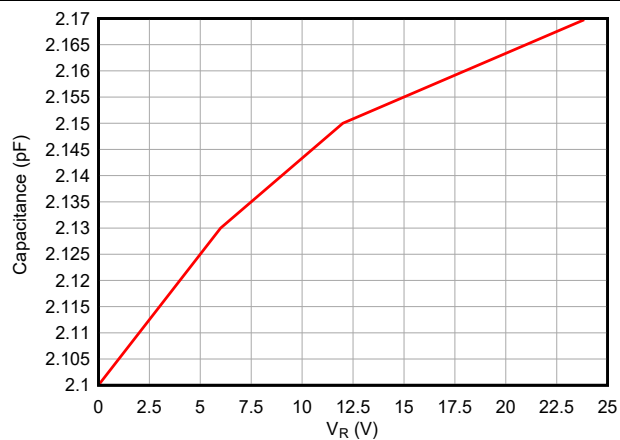
图 5-5. 电容与偏置电压间的关系
