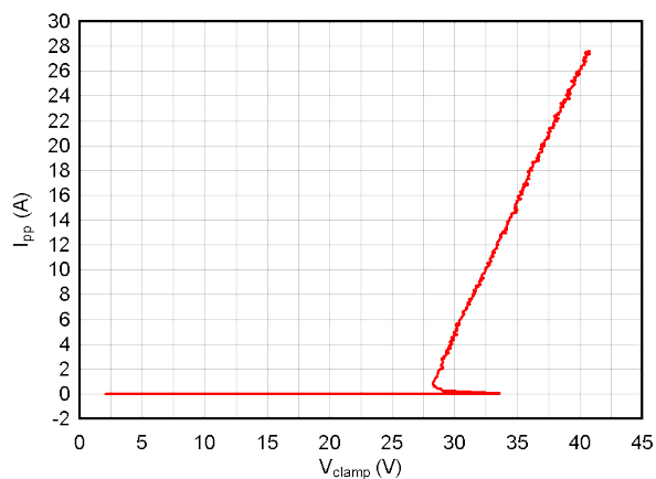
图 5-7. 正 TLP 曲线
