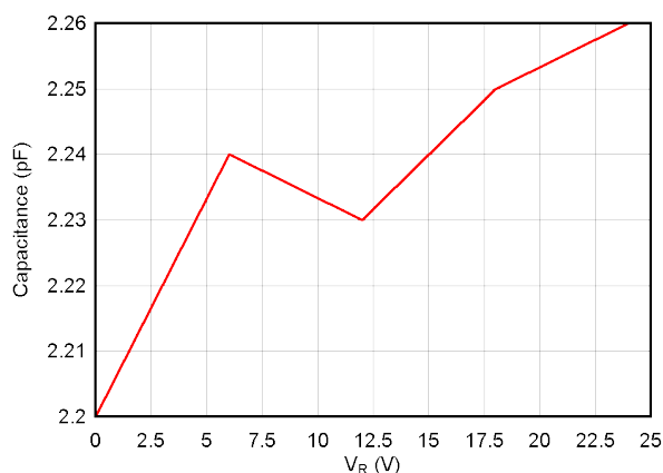
图 5-11. 电容与偏置电压间的关系
