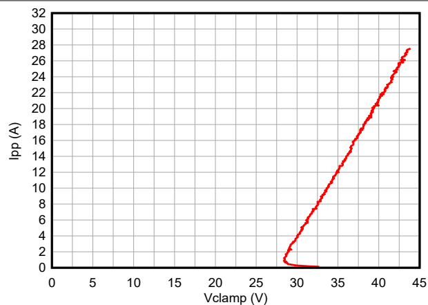
图 5-1. 正 TLP 曲线
