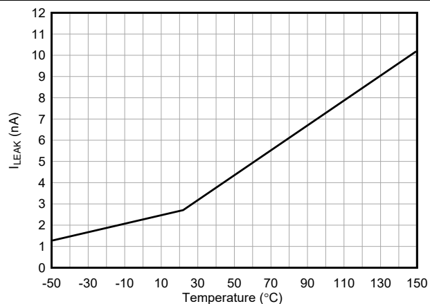
图 5-6. 漏电流与温度间的关系
