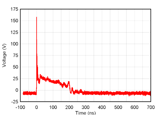
图 7-2. +8kV 钳位 IEC 波形
