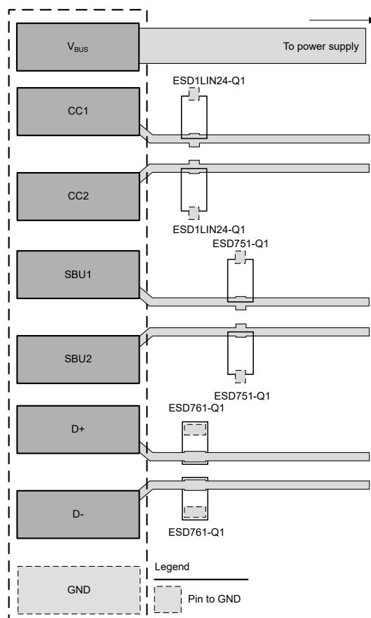
图 9-1. 布局建议
