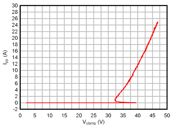
图 5-14. 负 TLP 曲线
