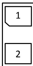
图 4-1. DPY 封装，2 引脚 X1SON ( 顶视图 )
