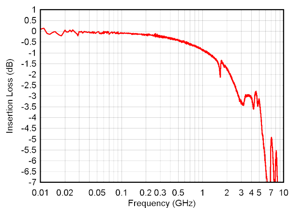
图 5-17. 插入损耗
