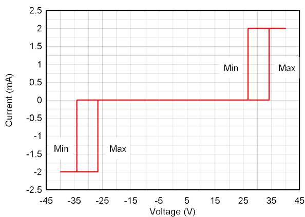
图 5-12. 直流电压扫描 I-V 曲线
