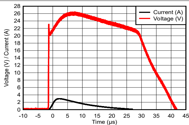
图 5-5. 8/20 \mu s 浪涌响应
