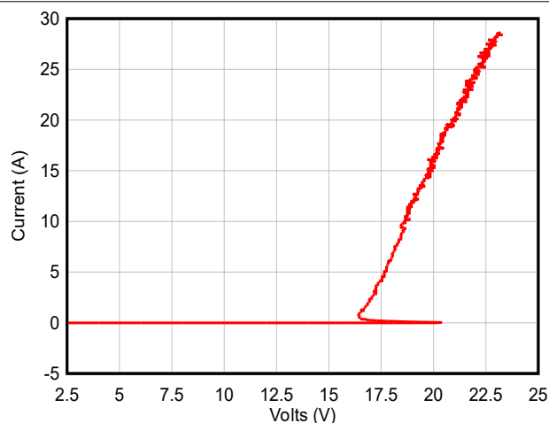
图 5-1. 正 TLP 曲线
