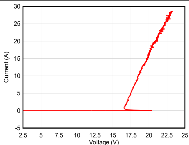
图 5-2. 负 TLP 曲线
