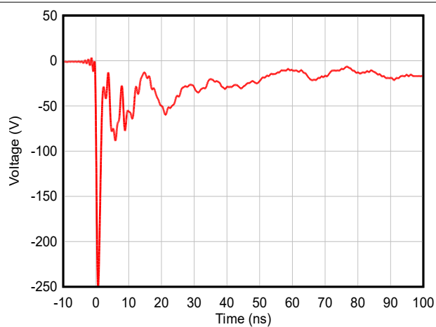
图 5-4. -8kV 钳位 IEC 波形
