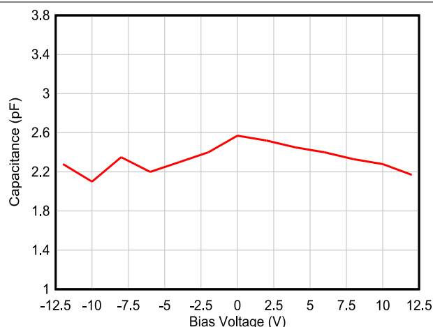
图 5-5. 电容与偏置电压之间的关系
