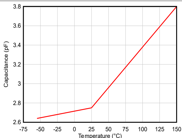
图 5-6. 电容与温度间的关系
