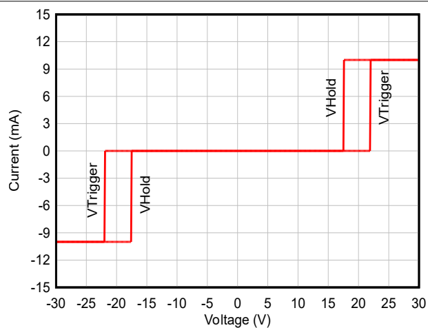
图 5-8. DC-IV 曲线
