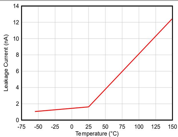
图 5-7. 漏电流与温度之间的关系
