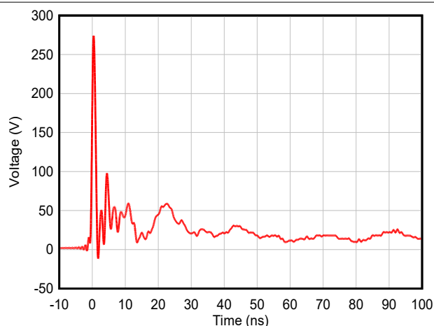
图 5-3. +8kV 钳位 IEC 波形
