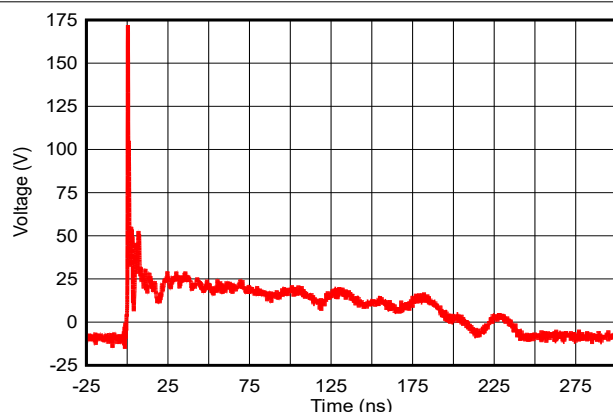
图 5-1. +8kV 钳位 IEC 波形
