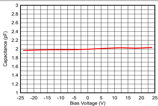
图 5-6. 偏置电压与电容间的关系
