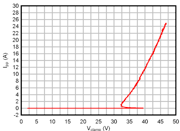
图 5-14. 负 TLP 曲线
