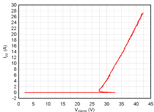
图 5-13. 正 TLP 曲线
