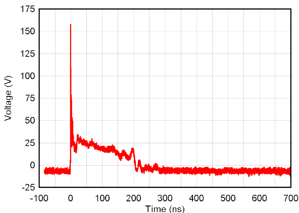
图 7-2. +8kV 钳位 IEC 波形
