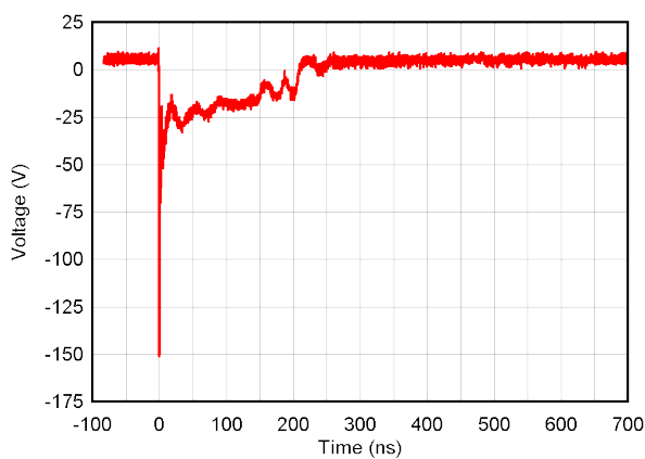
图 5-10. -8kV 钳位 IEC 波形
