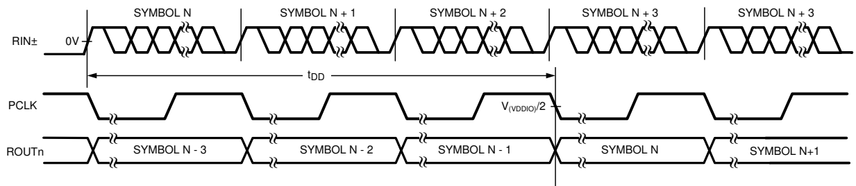
图 4-6. Deserializer Delay
