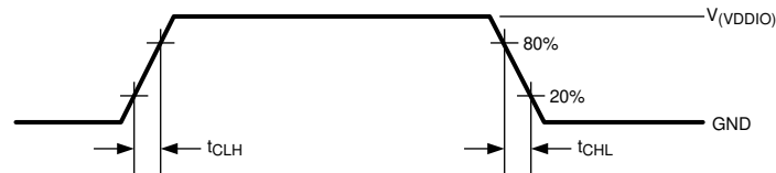
图 4-1. LVCMOS Transition Times
