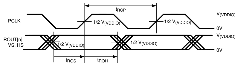
图 4-7. Deserializer Output Setup/Hold Times
