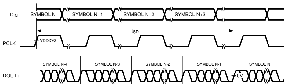
图 6-10. Serializer Delay
