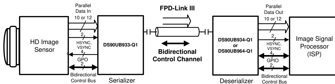
简化原理图
