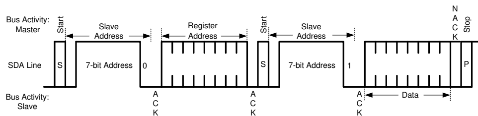
图 7-10. Read Byte
