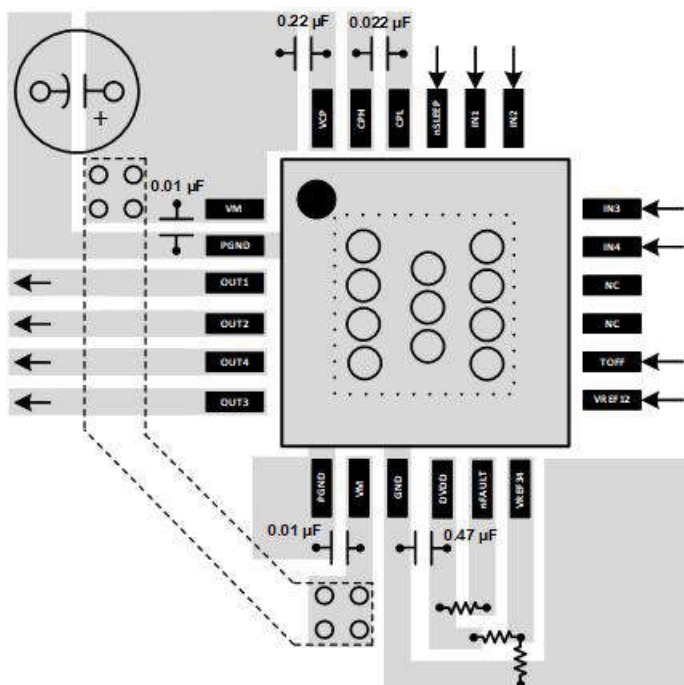
图 10-2. QFN 布局建议
