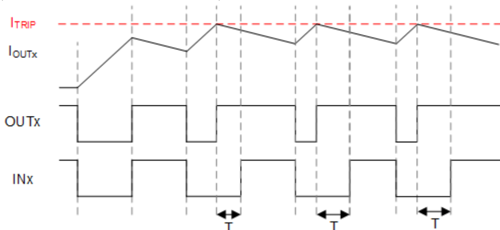
图 7-6. 电感负载连接至 VM，逐周期控制，T 必须短于 DRV8935 的 T_{OFF} 。
