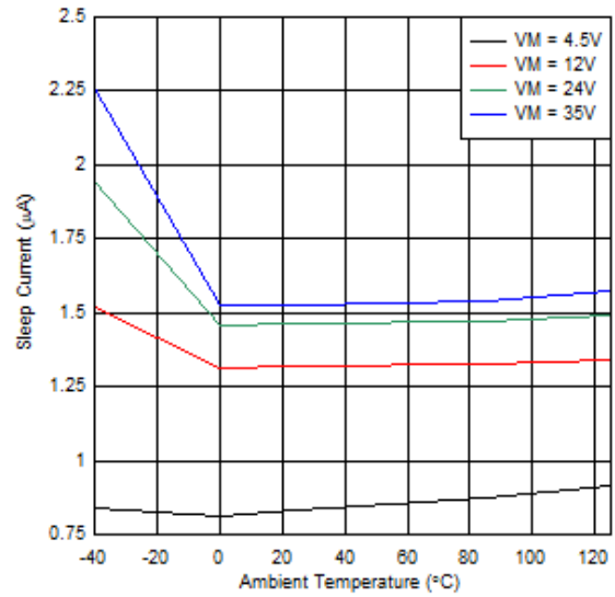
图 6-2. 睡眠电流与温度间的关系
