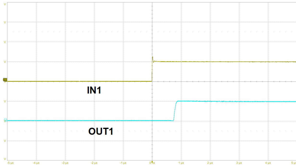
图 8-3. IN1 至 OUT1 传播延迟
