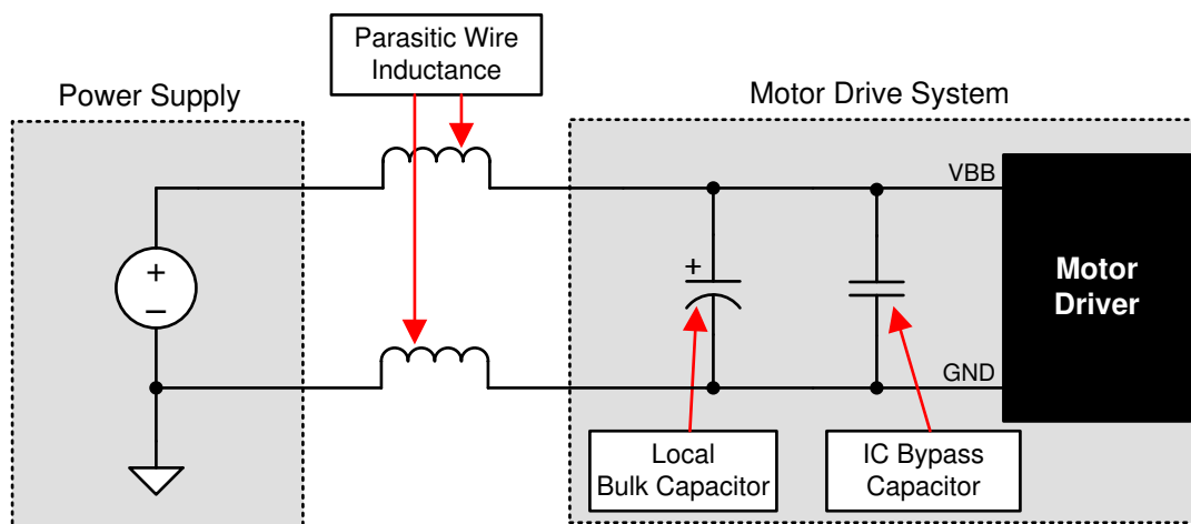
图 9-1. 系统电源寄生效应示例
