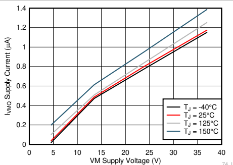
图 6-2. 睡眠电流 ( I_{VMQ} ) 与电源电压 ( V_{VM} ) 间的关系
