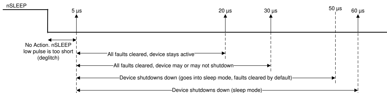
图 7-14. nSLEEP Reset Pulse
