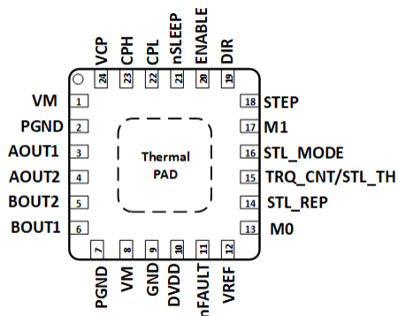
图 5-2. RGE 封装 24 引脚 VQFN (带有外露散热焊盘) 俯视图
