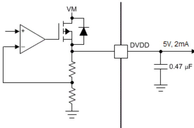
图 7-7. 线性稳压器方框图
