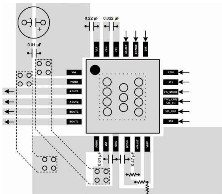
图 10-2. QFN 布局示例
