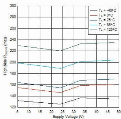
图 6-8. 高侧 R_{DS(ON)} 与电源电压间的关系
