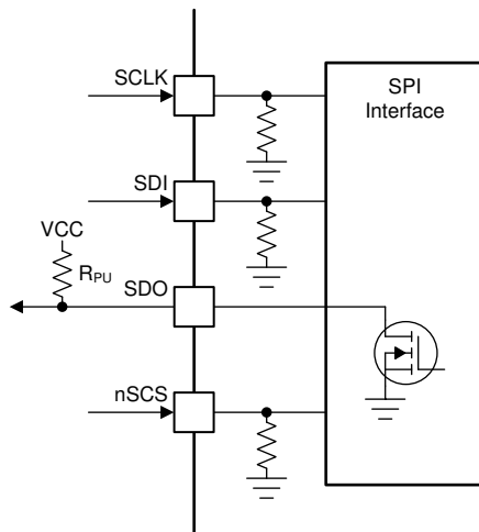
图 27. SPI
