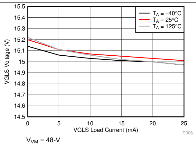
图 7. VGLS Voltage Over Load Current
