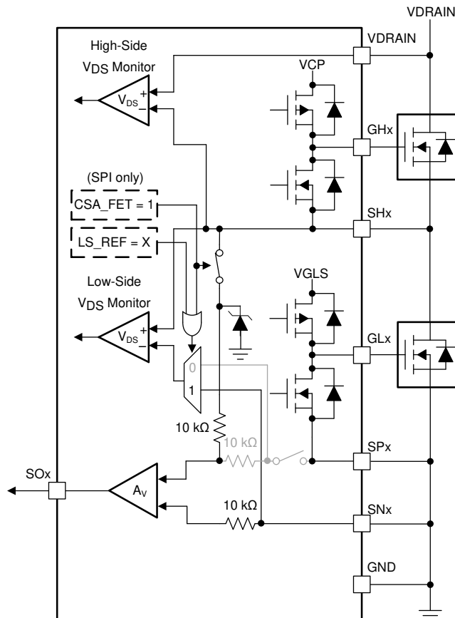
图 49. V_{DS} Sense Configuration
