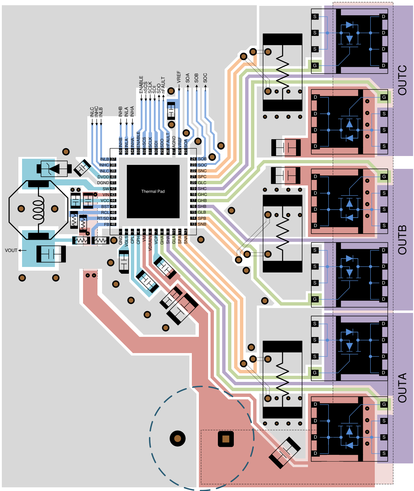
图 75. Layout Example
