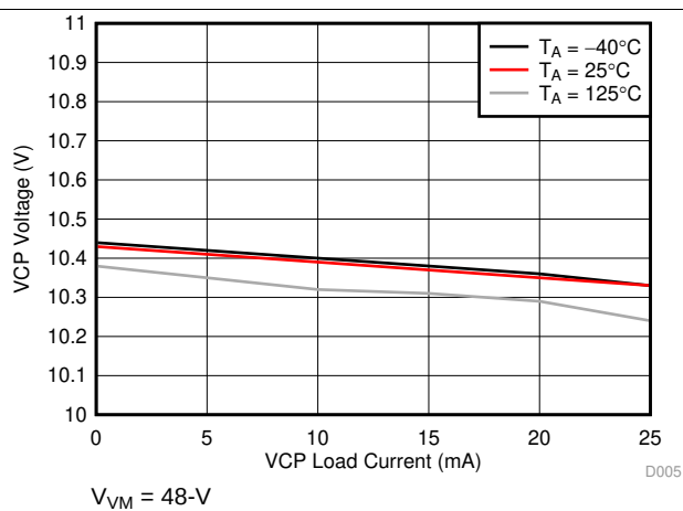
图 6. VCP Voltage Over Load
