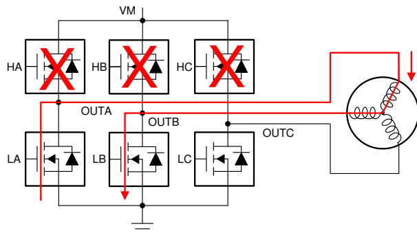
图 8-37. Brake State
