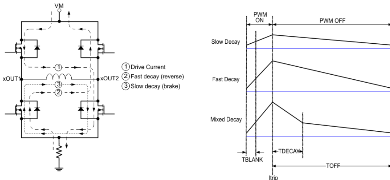
图 7-4. 衰减模式
