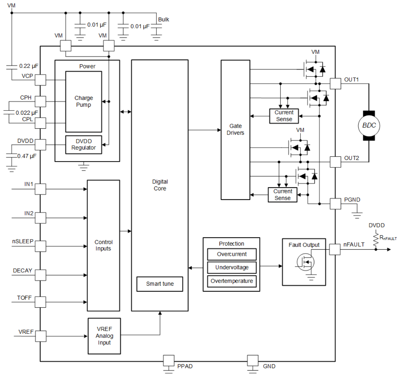
图 7-2. DRV8256P 方框图
