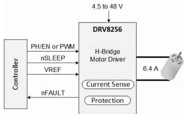
DRV8256 简化版原理图
