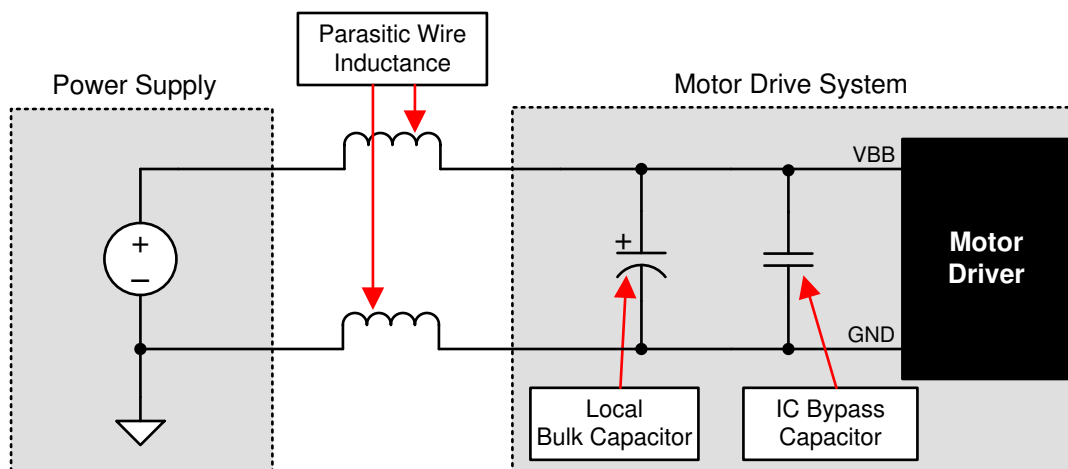
图 9-5. 带外部电源的电机驱动系统示例设置
