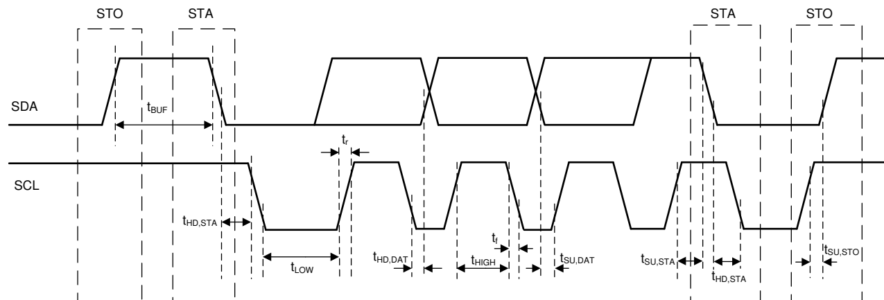
图 6-2. I²C 时序图
