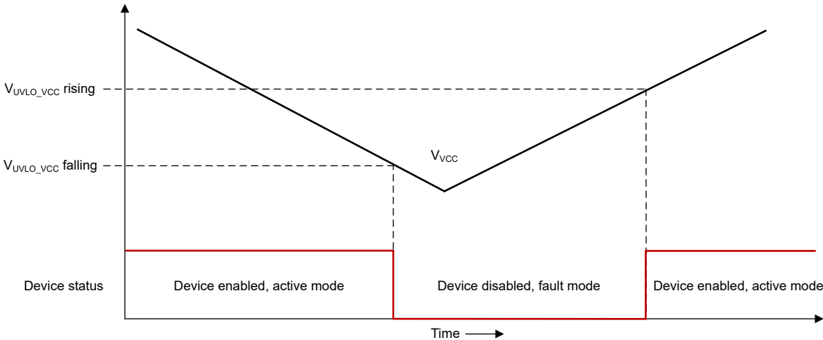
图 7-14. UVLO 运行
