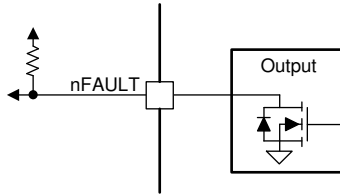
图 7-15. nFAULT 引脚
