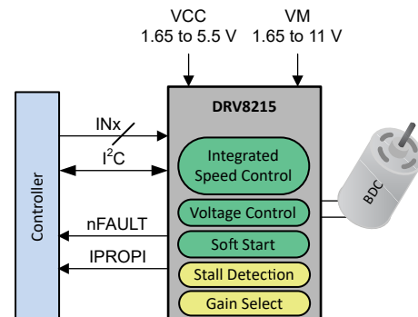
简化原理图
