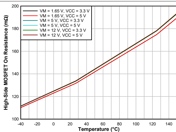
图 6-3. 高侧 MOSFET 导通电阻 (mΩ)
