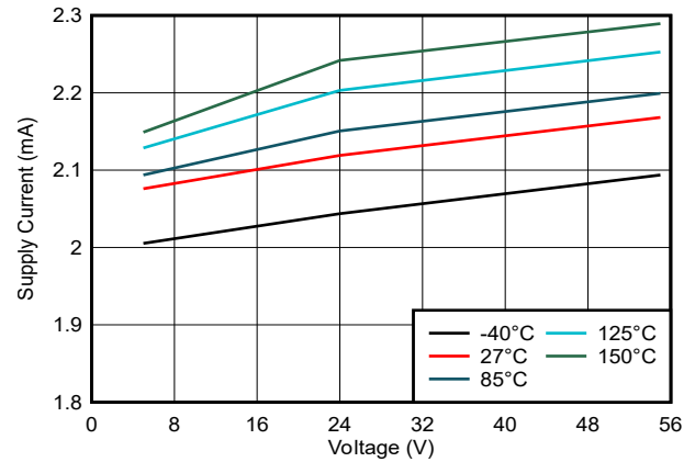
图 5-3. 电源电流与 V_M 间的关系
