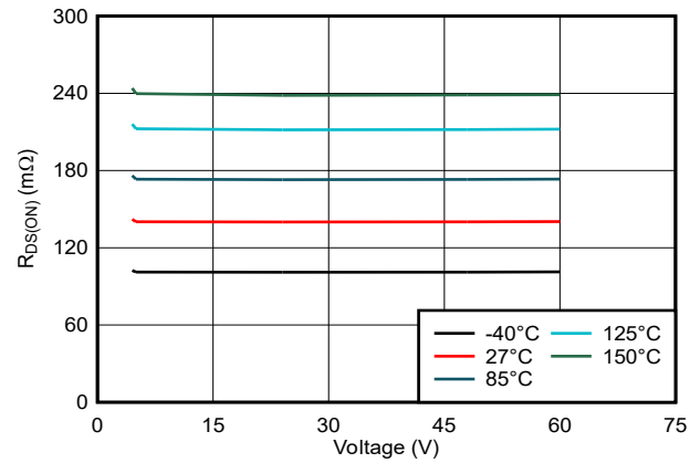
图 5-5. R_{DS(on)} 与 V_M 间的关系
